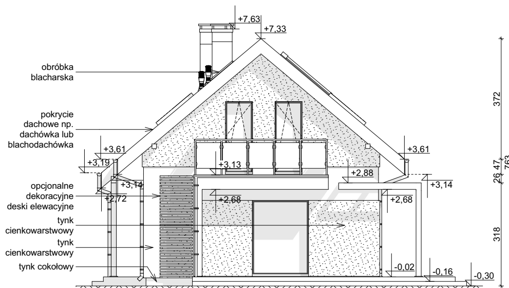
ELEWACJA BOCZNA
