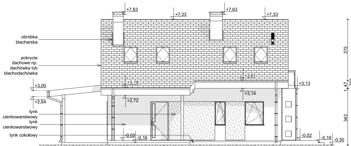
ELEWACJA FRONTOWA
