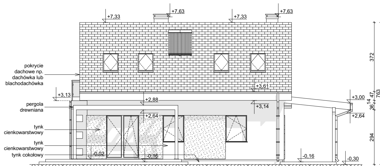
ELEWACJA OGRODOWA
