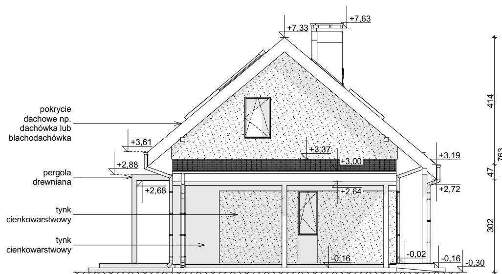
ELEWACJA BOCZNA
