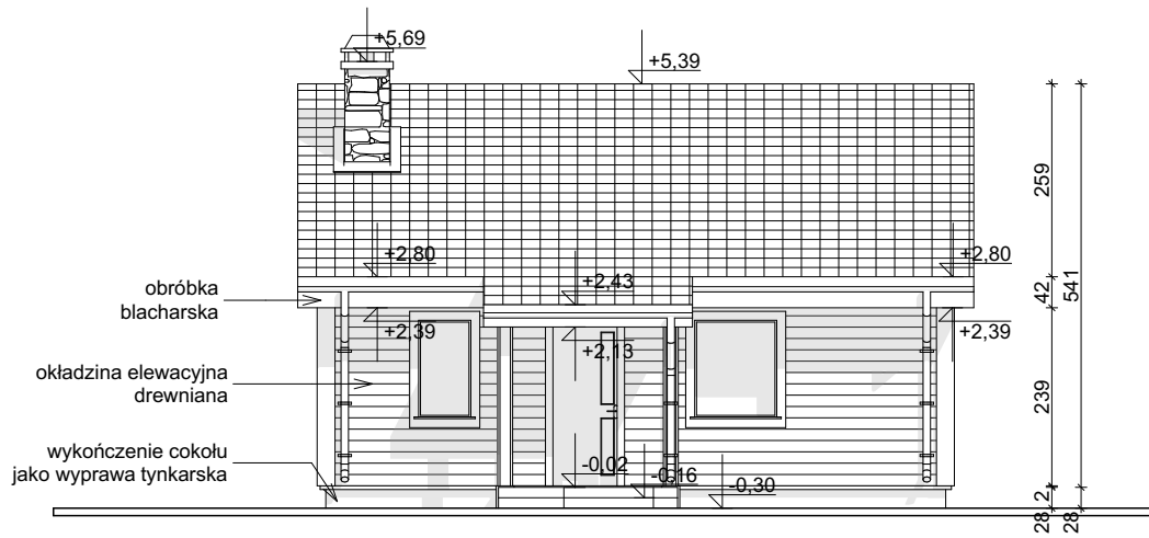
ELEWACJA FRONTOWA
