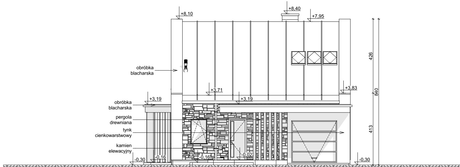
ELEWACJA FRONTOWA
