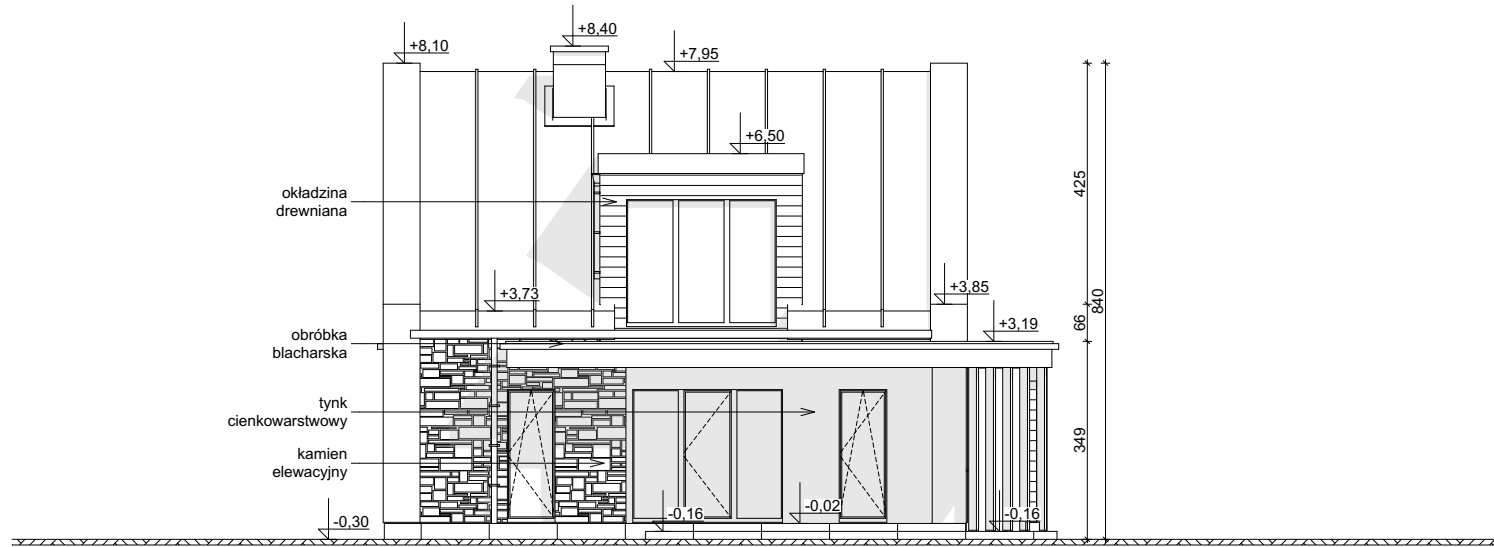
ELEWACJA OGRODOWA
