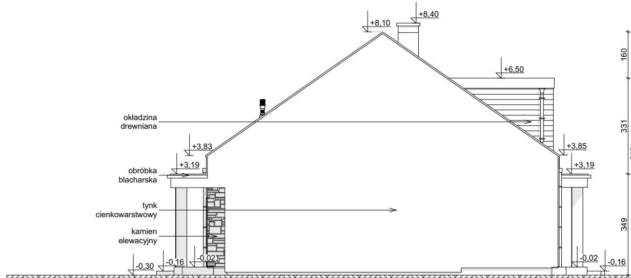
ELEWACJA BOCZNA
