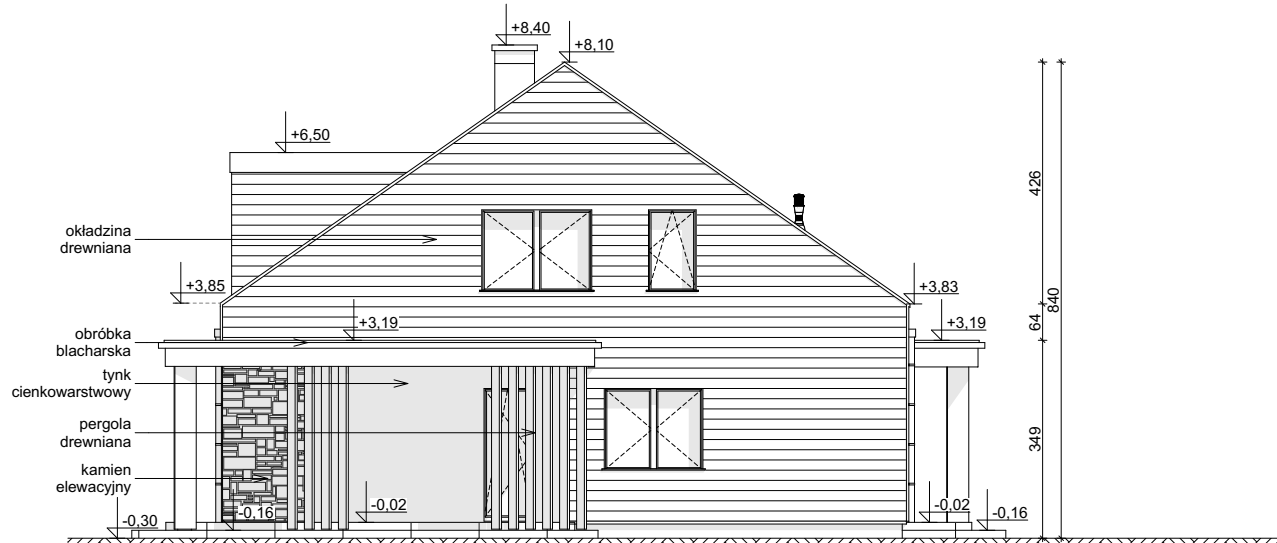
ELEWACJA BOCZNA
