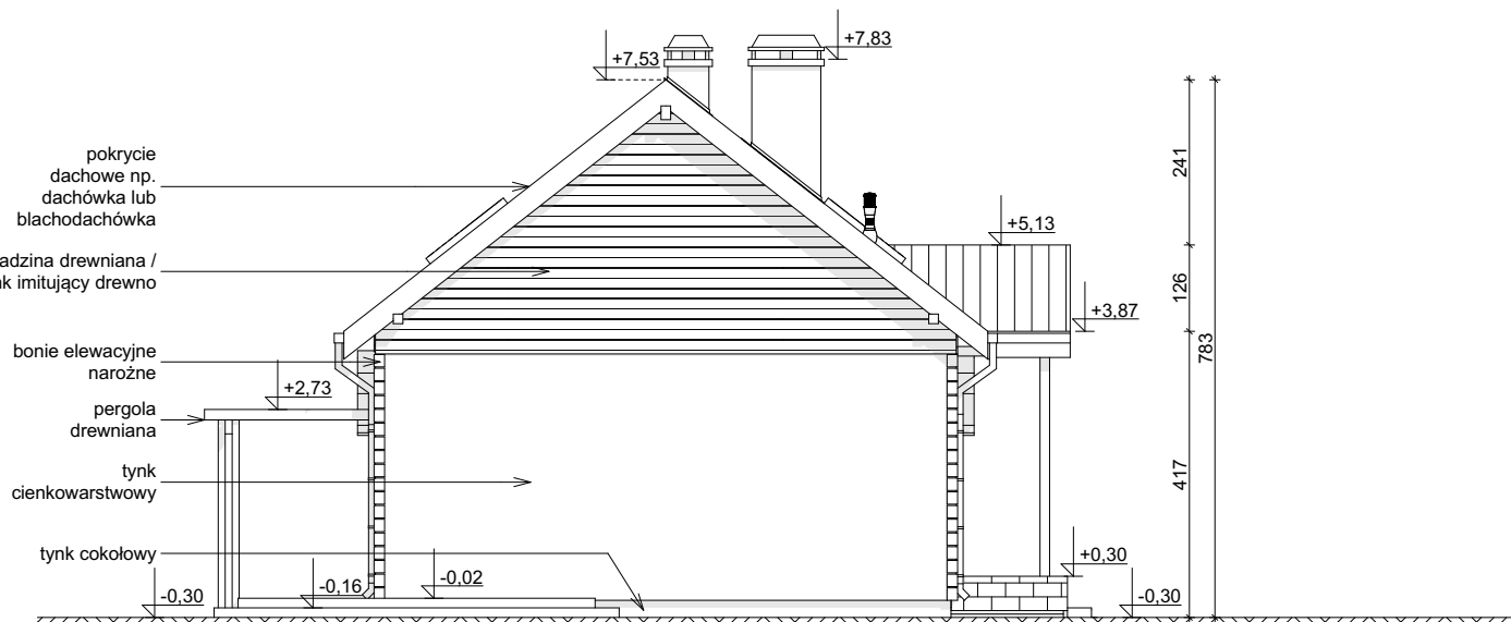
ELEWACJA BOCZNA
