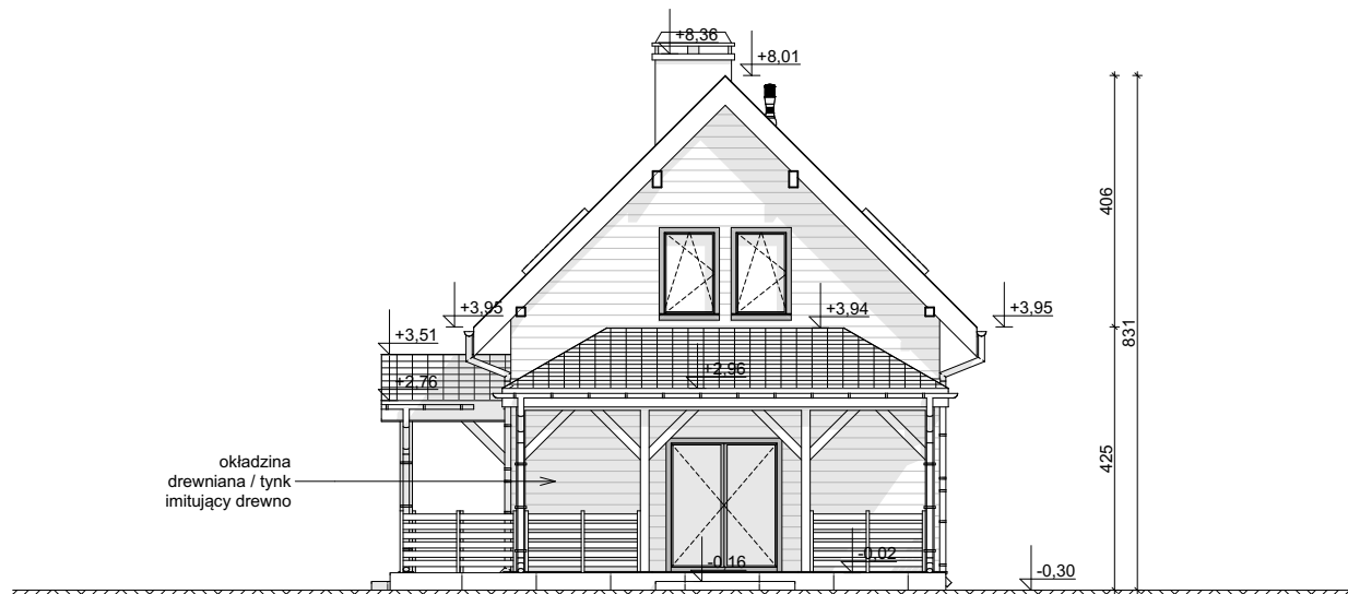
ELEWACJA BOCZNA
