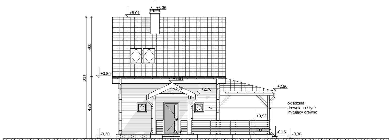
ELEVACJA FRONTOWA
