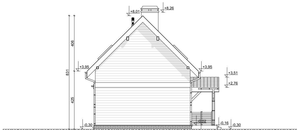
ELEVACJA BOCZNA
