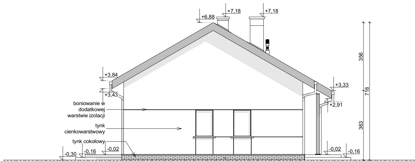
ELEWACJA BOCZNA
