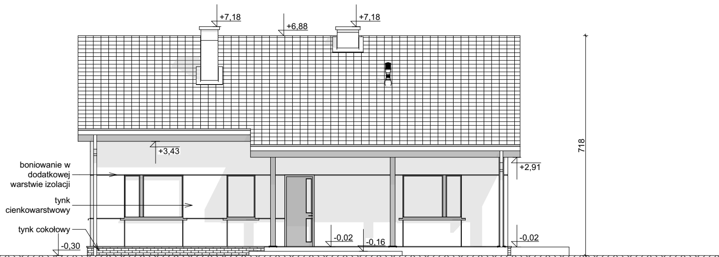
ELEWACJA FRONTOWA
