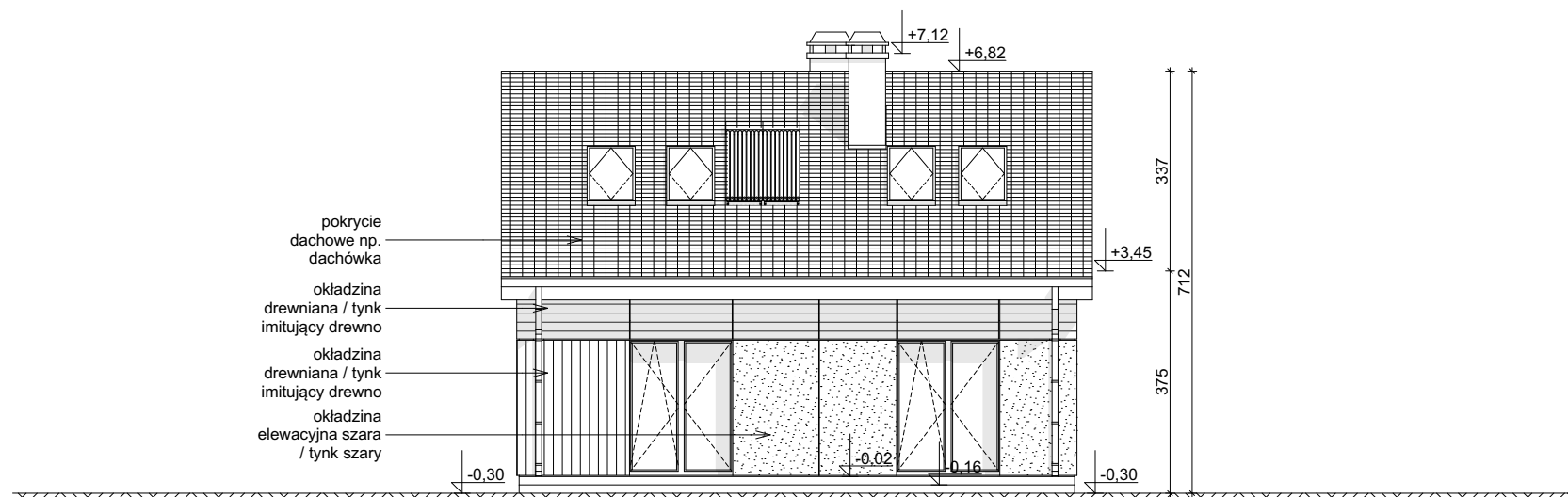
ELEWACJA OGRODOWA
