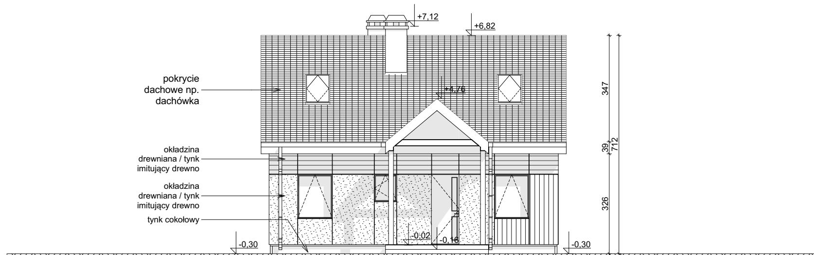
ELEWACJA FRONTOWA
