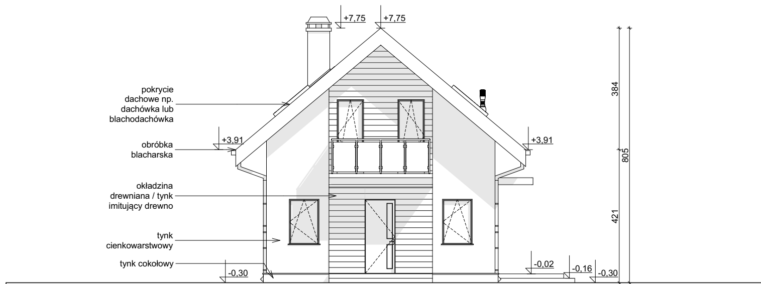
ELEWACJA FRONTOWA
