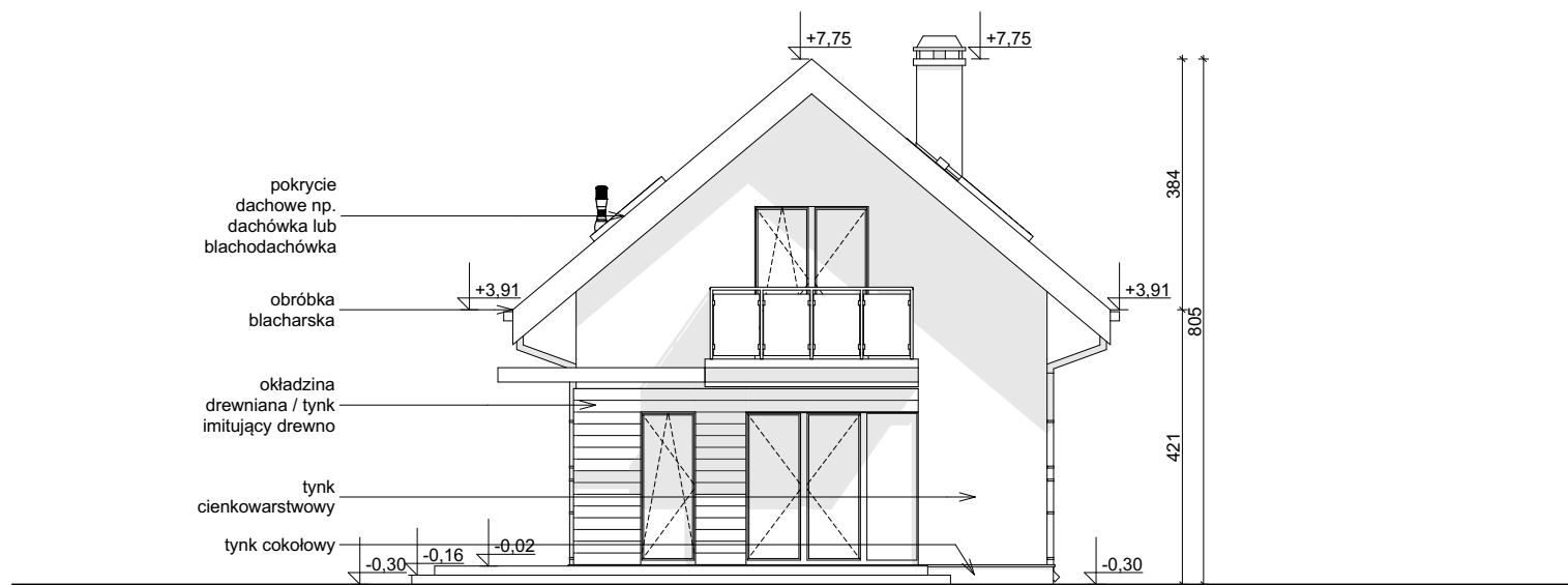
ELEWACJA OGRODOWA
