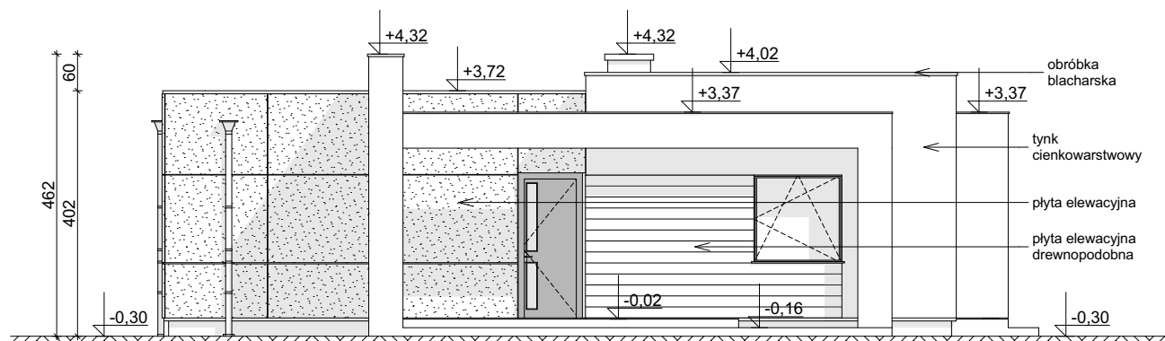
ELEWACJA FRONTOWA
