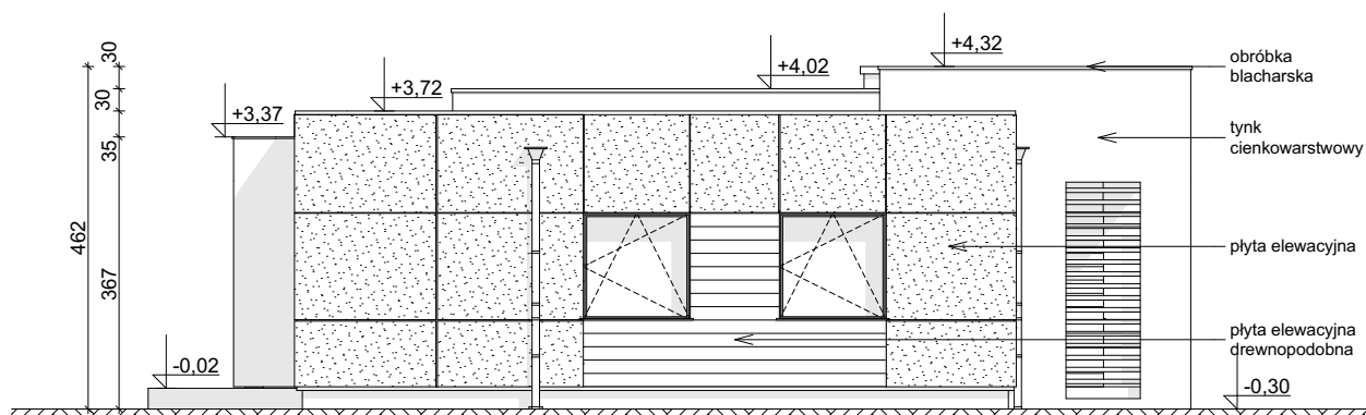
ELEWACJA BOCZNA
