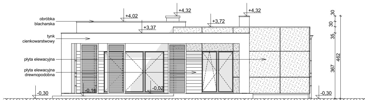
ELEWACJA OGRODOWA
