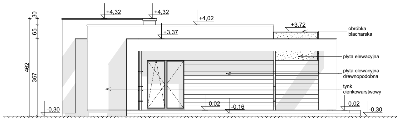
ELEWACJA BOCZNA
