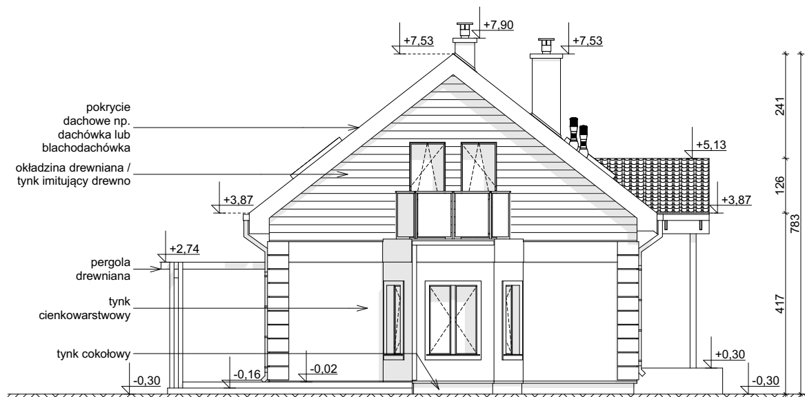
ELEWACJA BOCZNA
