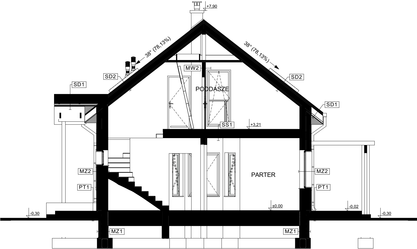
PRZEKRÓJ B-B
