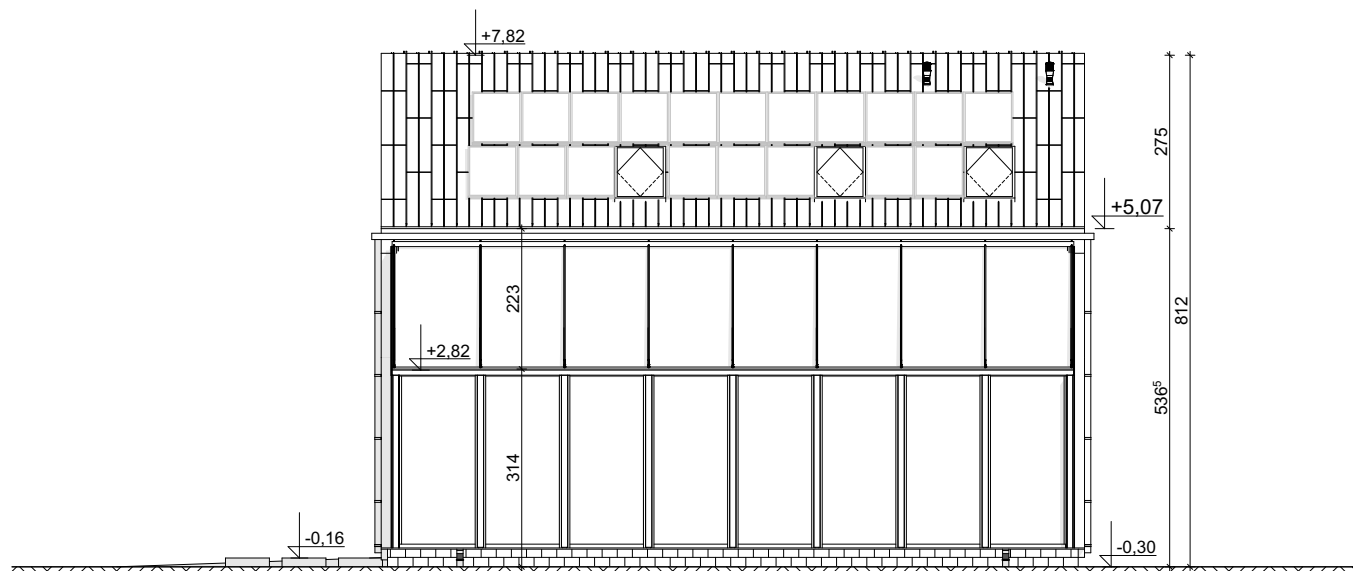
ELEWACJA BOCZNA
