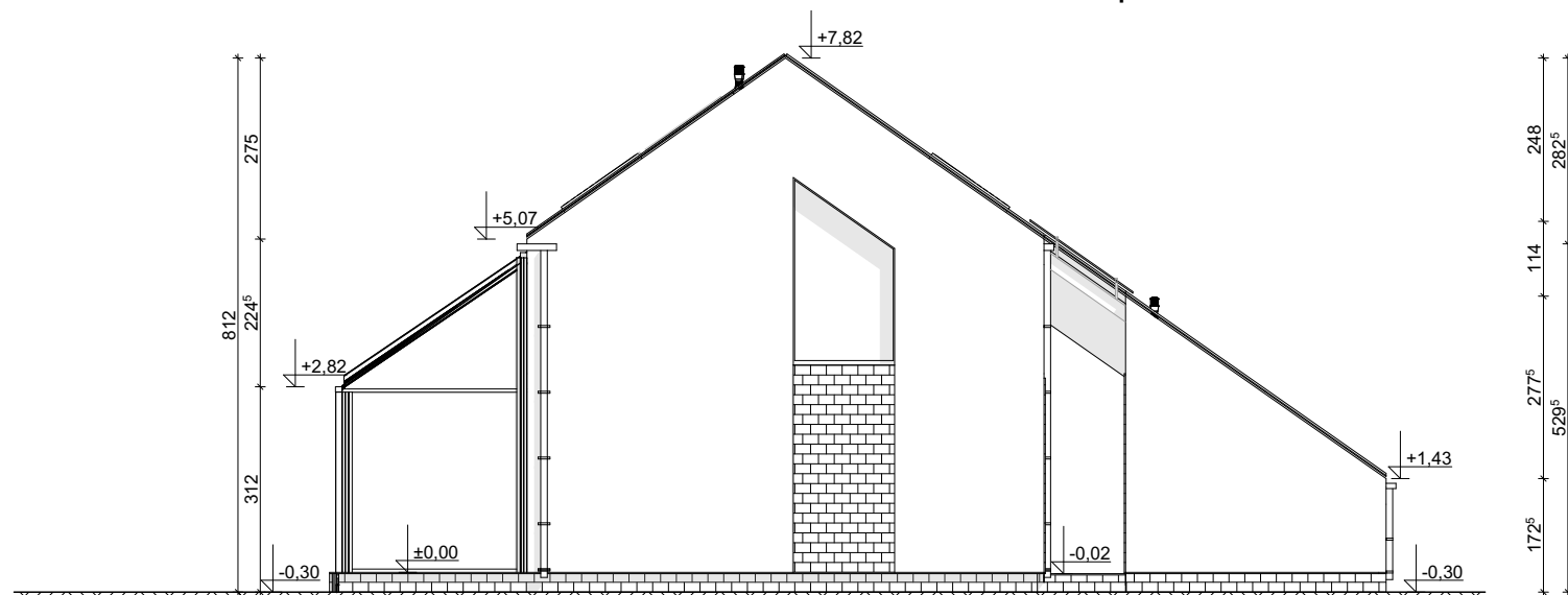
ELEWACJA TYLNA
