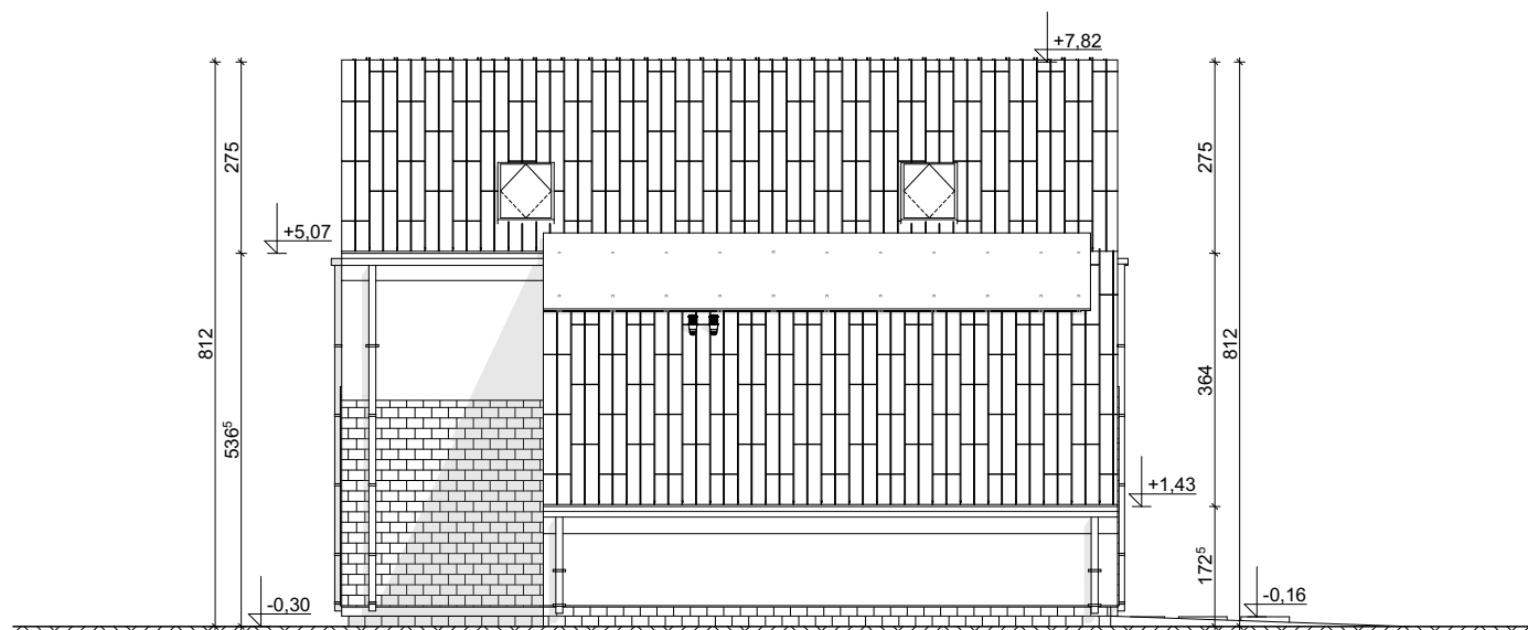
ELEWACJA BOCZNA
