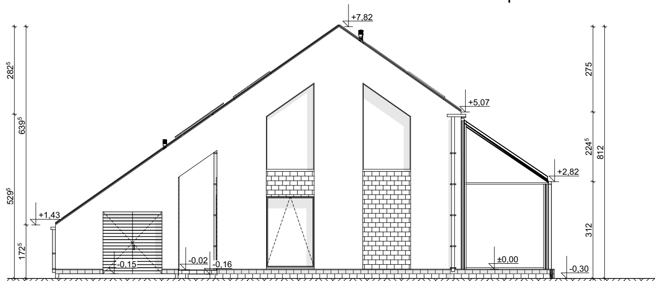
ELEWACJA FRONTOWA
