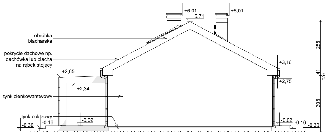
ELEWACJA BOCZNA
