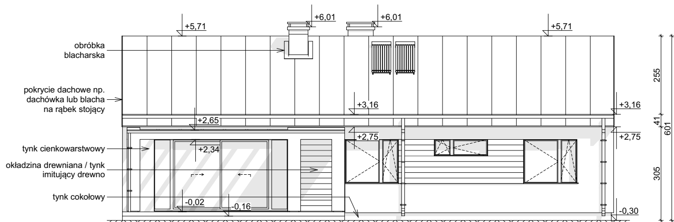
ELEWACJA OGRODOWA
