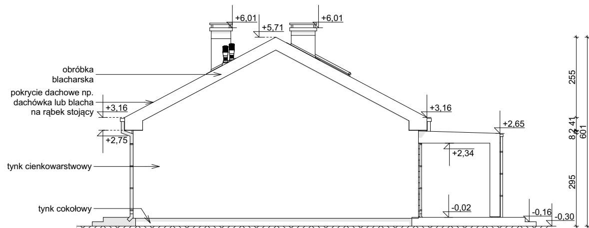
ELEWACJA BOCZNA
