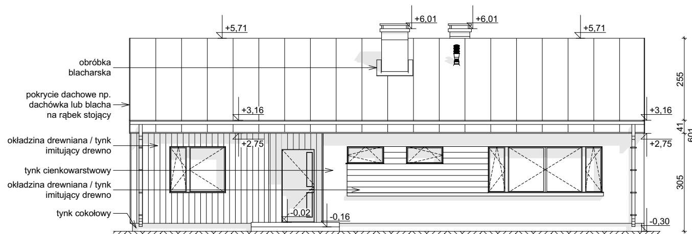
ELEWACJA FRONTOWA
