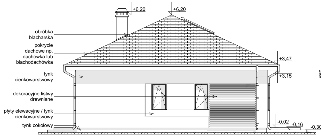
ELEWACJA BOCZNA
