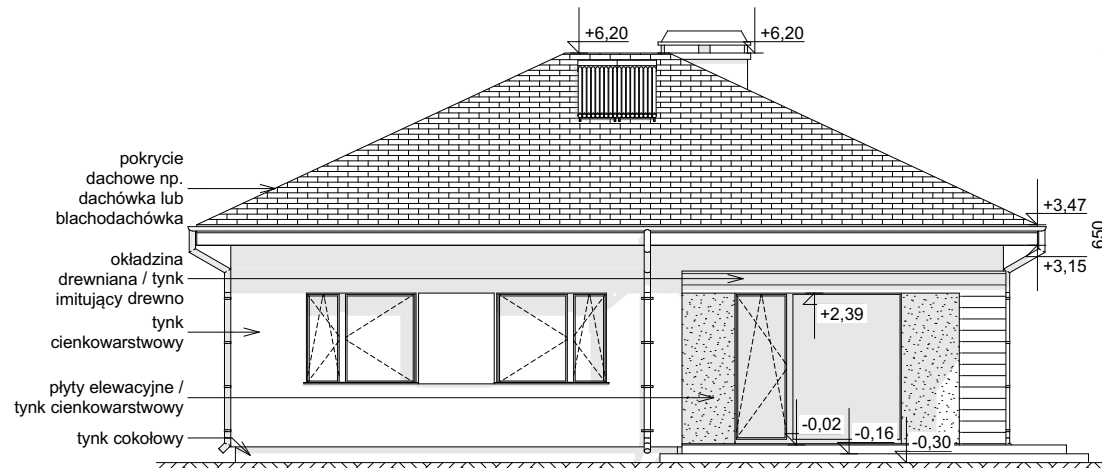
ELEWACJA OGRODOWA
