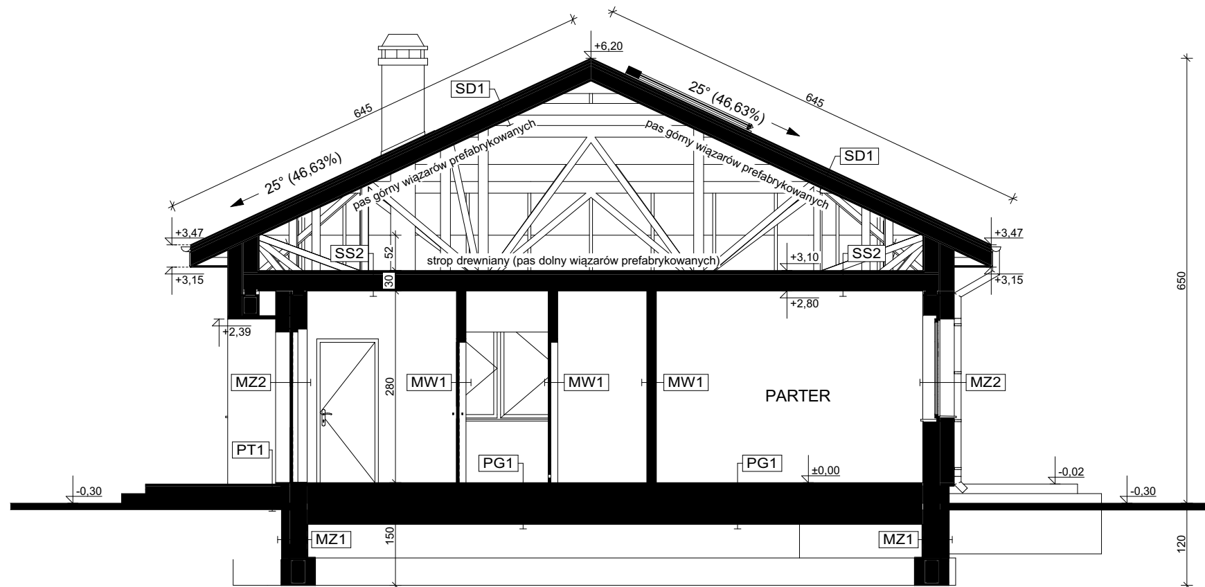
PRZEKRÓJ B-B
