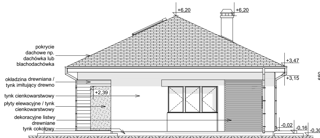
ELEWACJA BOCZNA
