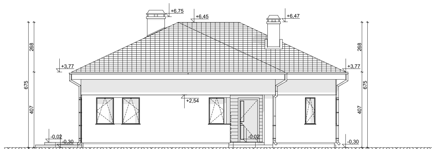
ELEVACJA FRONTOWA
