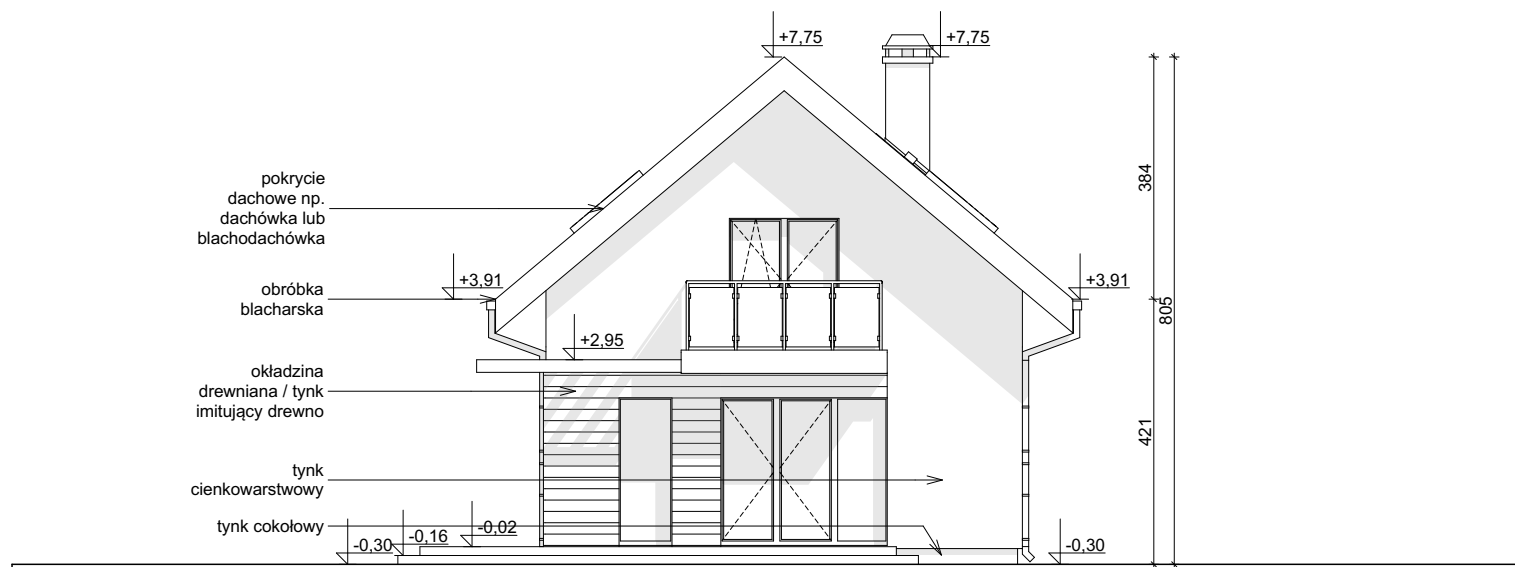
ELEWACJA OGRODOWA
