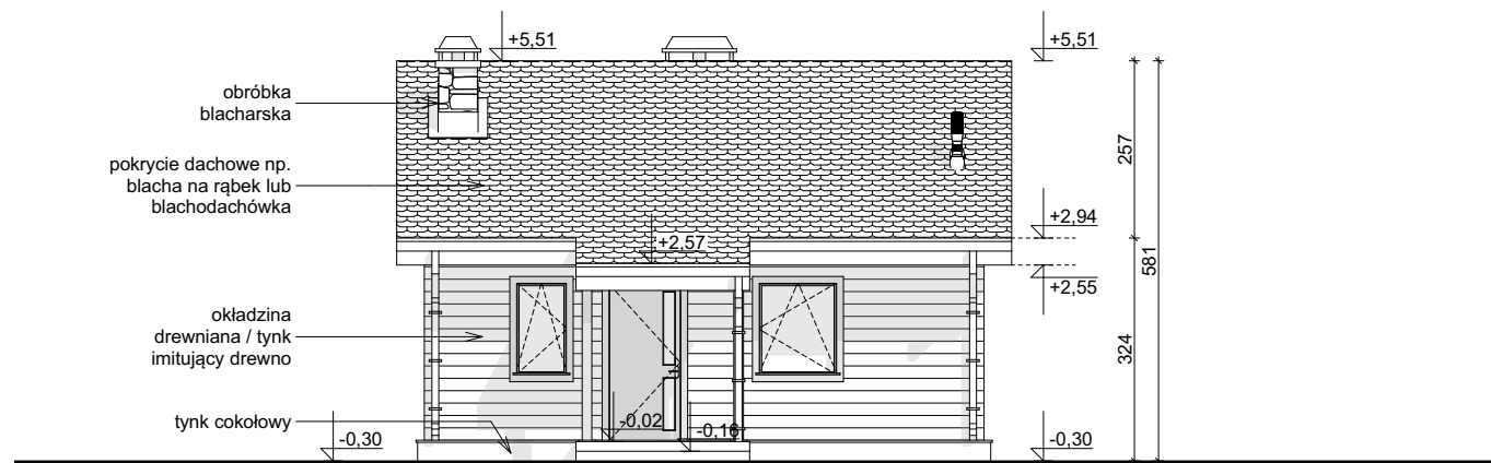
ELEWACJA FRONTOWA
