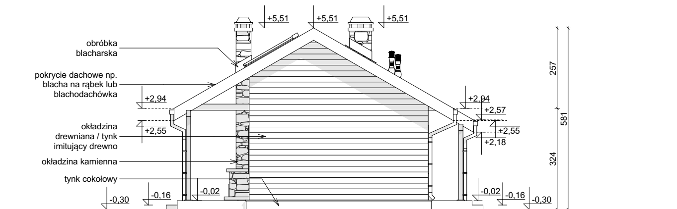
ELEWACJA BOCZNA
