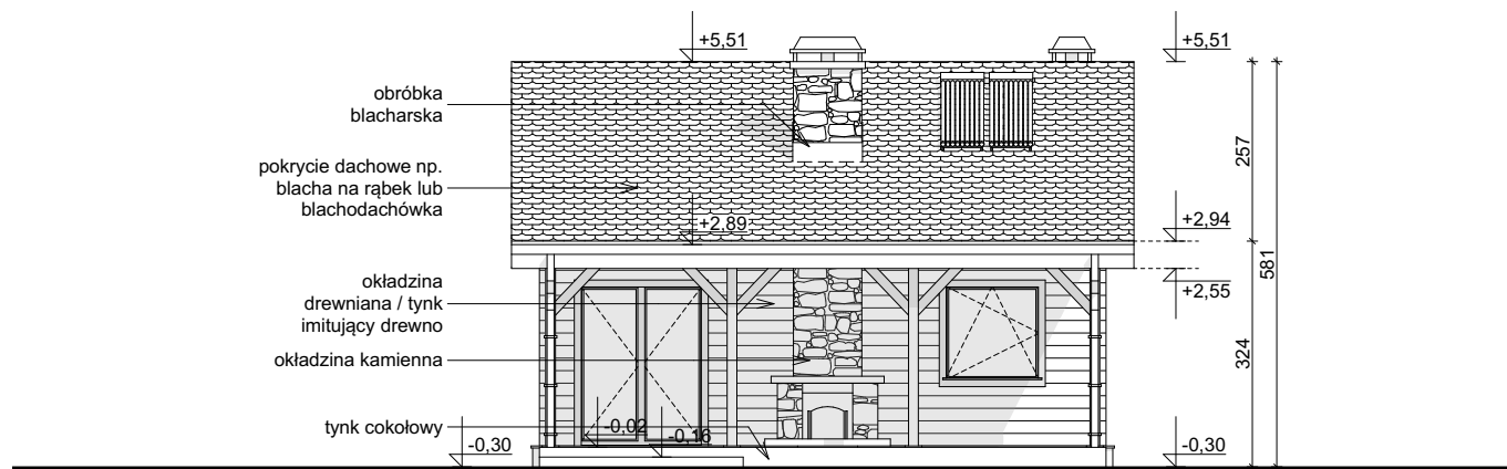
ELEWACJA OGRODOWA
