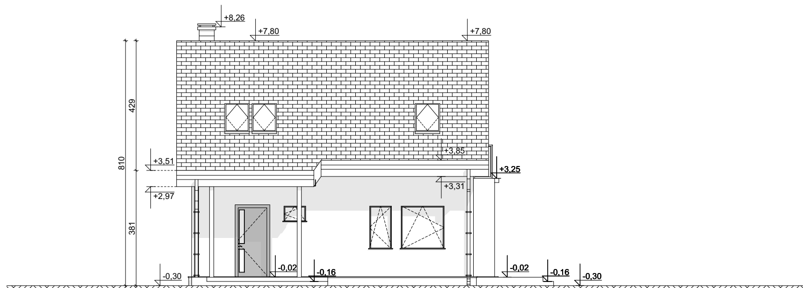
ELEWACJA FRONTOWA
