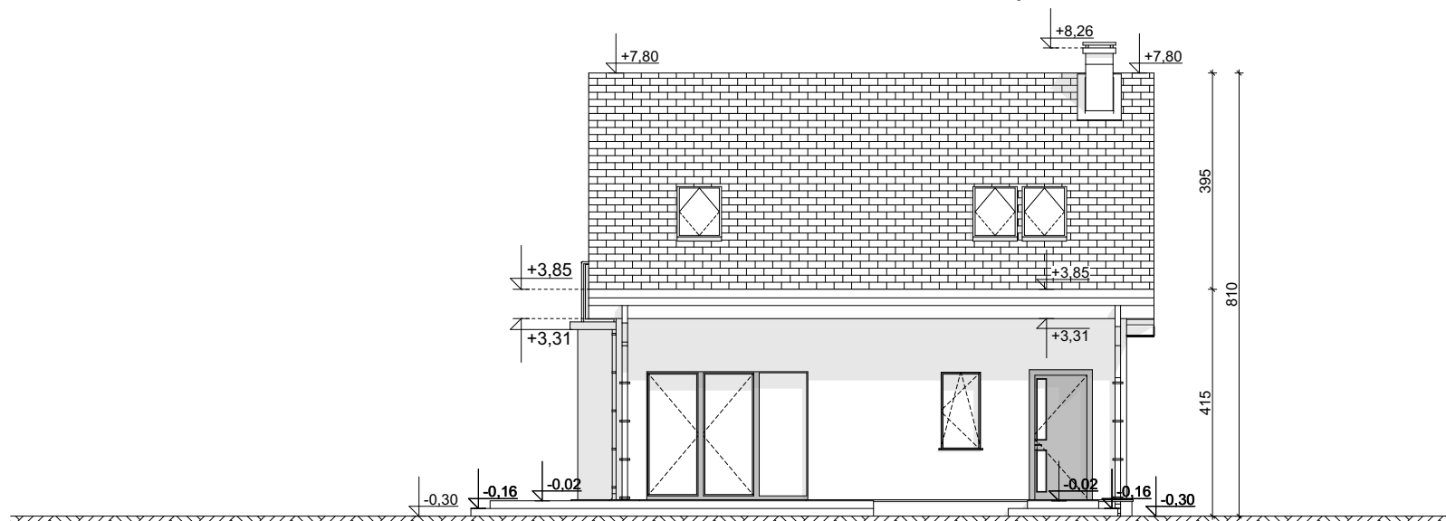
ELEWACJA OGRODOWA
