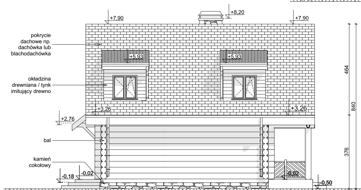
ELEWACJA BOCZNA
