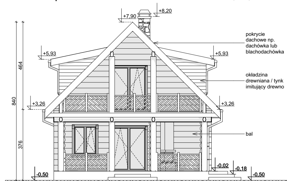
ELEWACJA OGRODOWA
