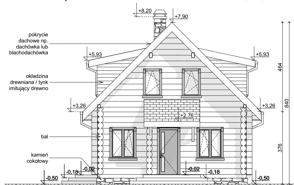
ELEVACJA FRONTOWA
