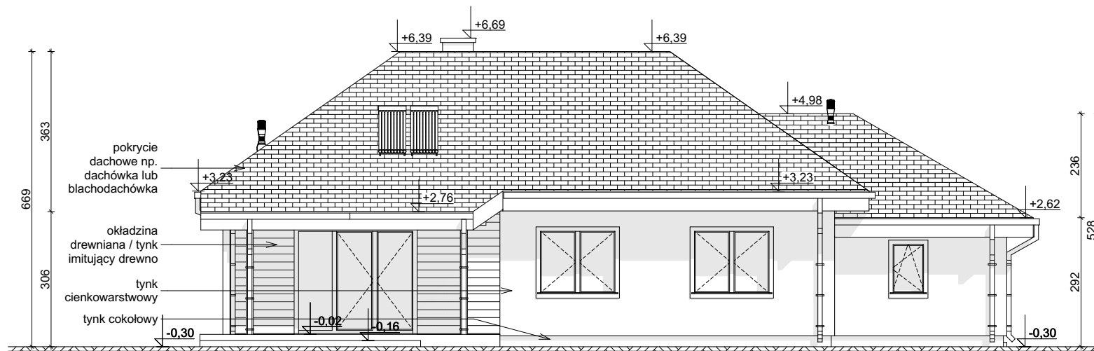
ELEWACJA OGRODOWA
