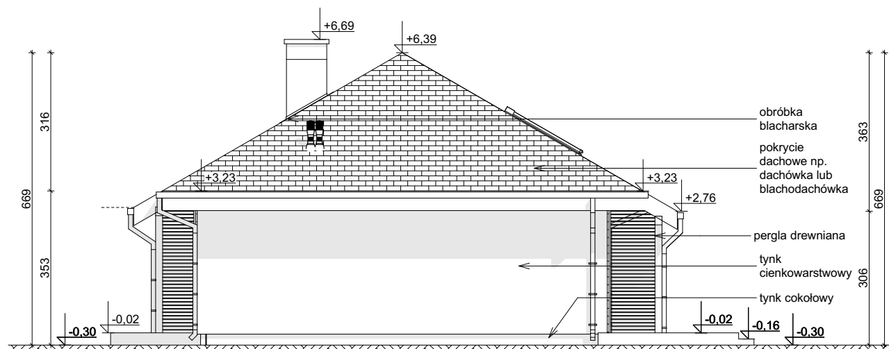
ELEWACJA BOCZNA
