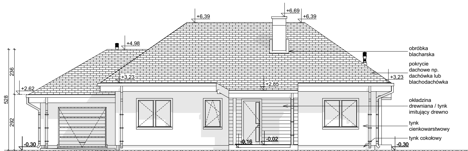
ELEWACJA FRONTOWA
