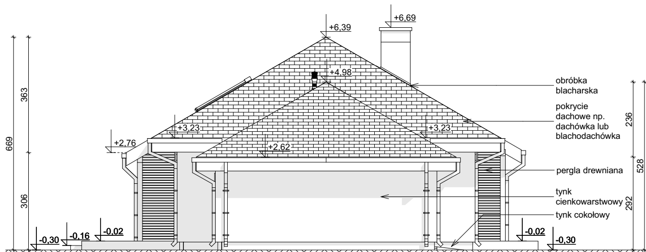
ELEWACJA BOCZNA
