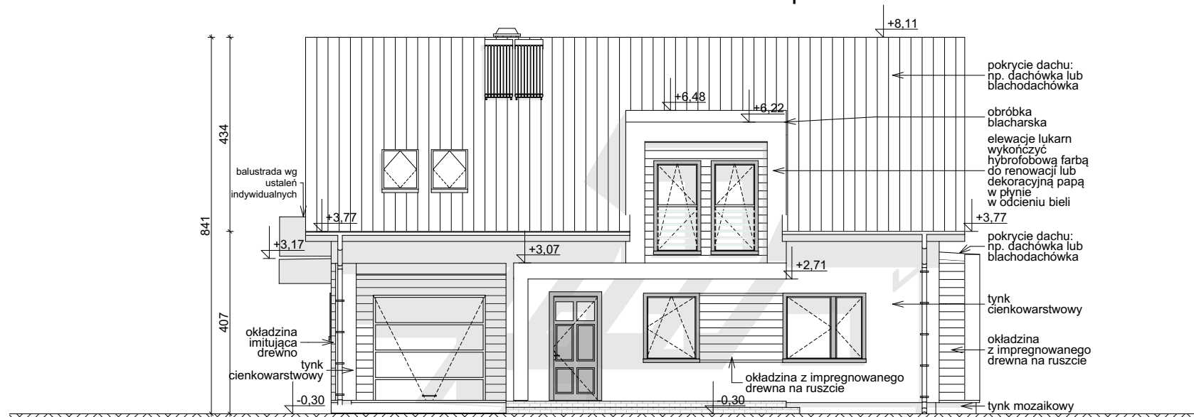
ELEWACJA FRONTOWA
