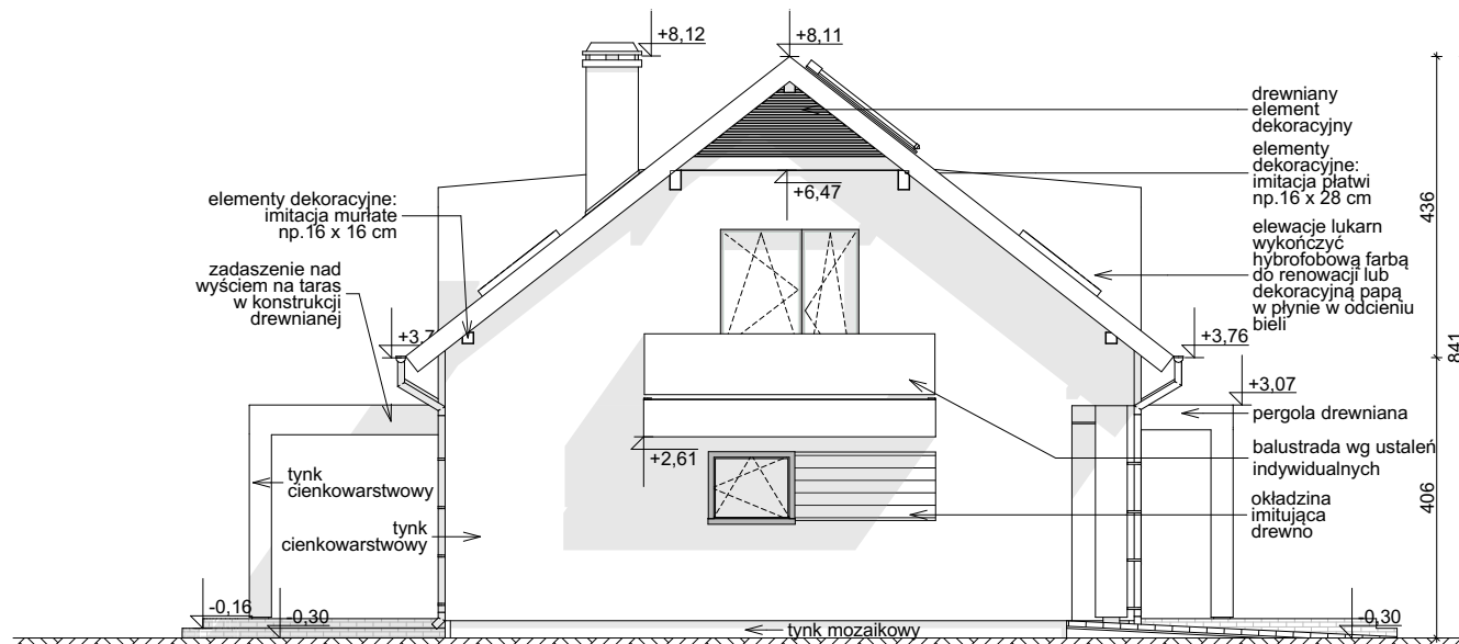
ELEWACJA BOCZNA
