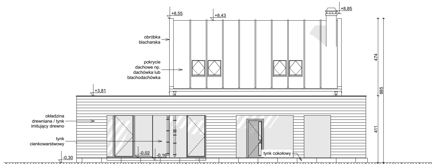
ELEWACJA OGRODOWA
