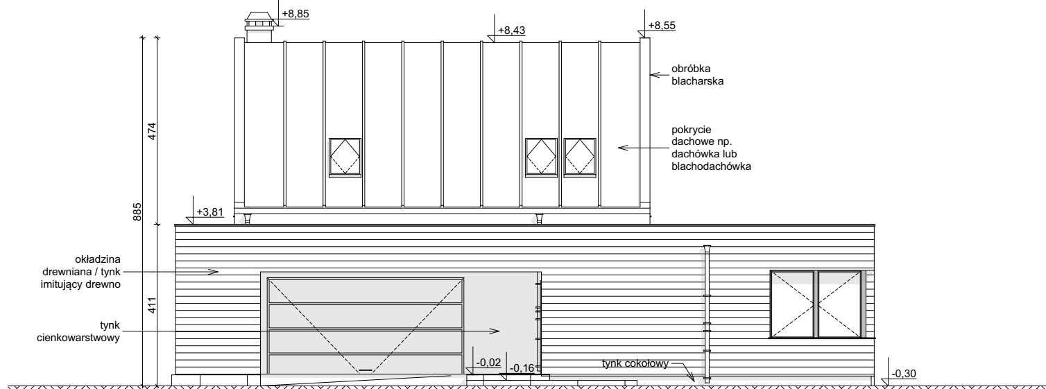
ELEWACJA FRONTOWA
