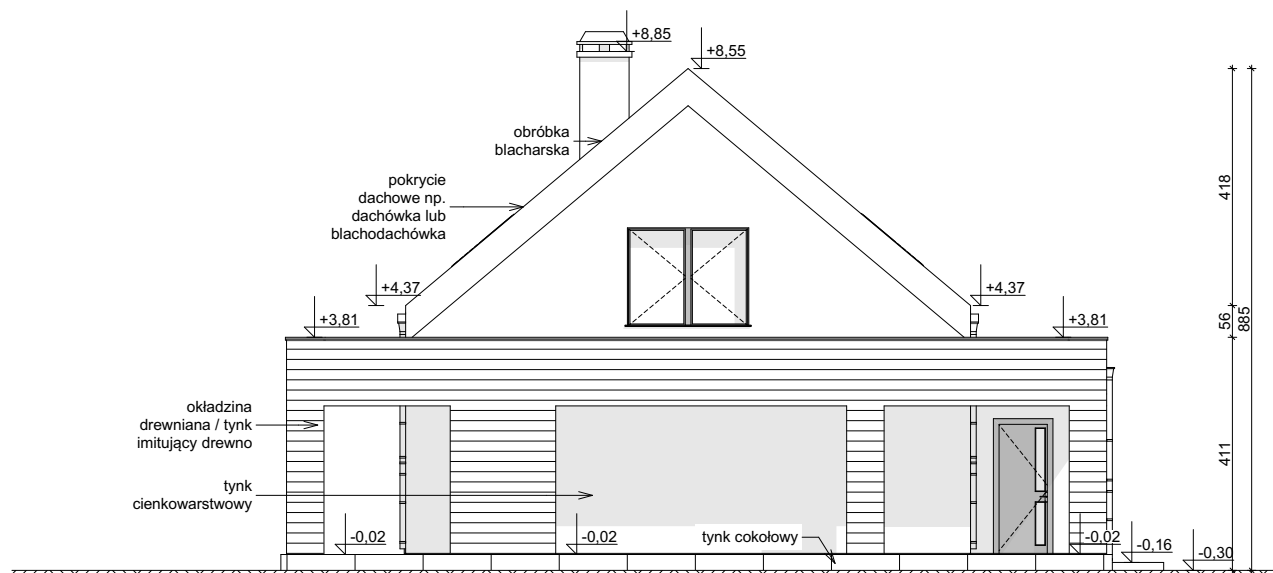
ELEWACJA BOCZNA
