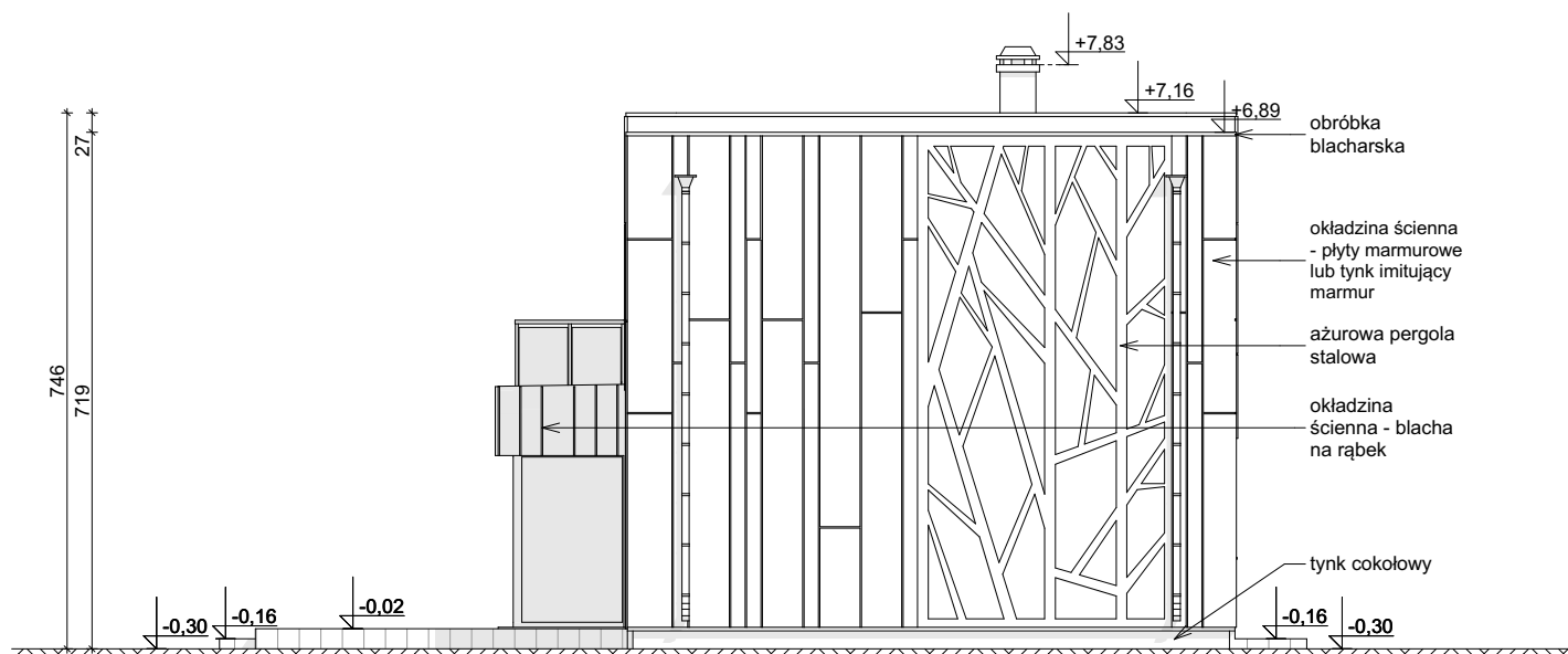
ELEWACJA BOCZNA
