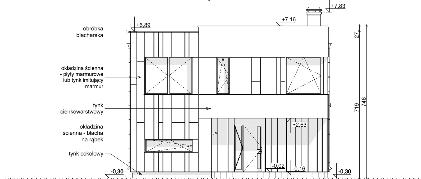
ELEWACJA FRONTOWA
