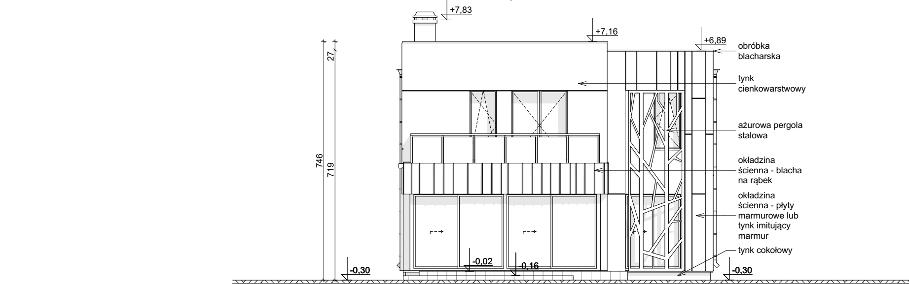
ELEWACJA OGRODOWA
