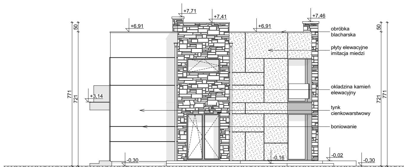
ELEVACJA BOCZNA
