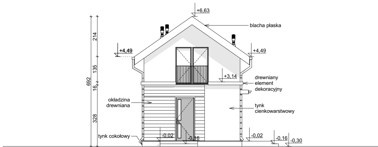
ELEWACJA FRONTOWA
