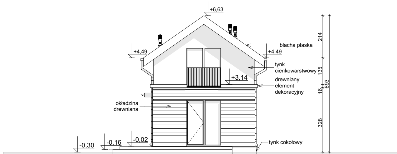
ELEWACJA OGRODOWA
