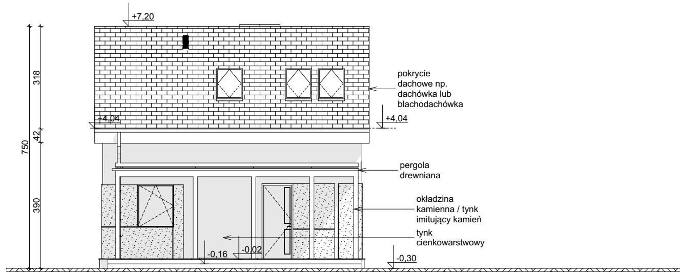
ELEWACJA FRONTOWA
