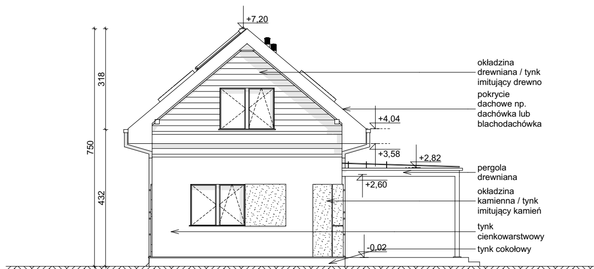
ELEWACJA BOCZNA
