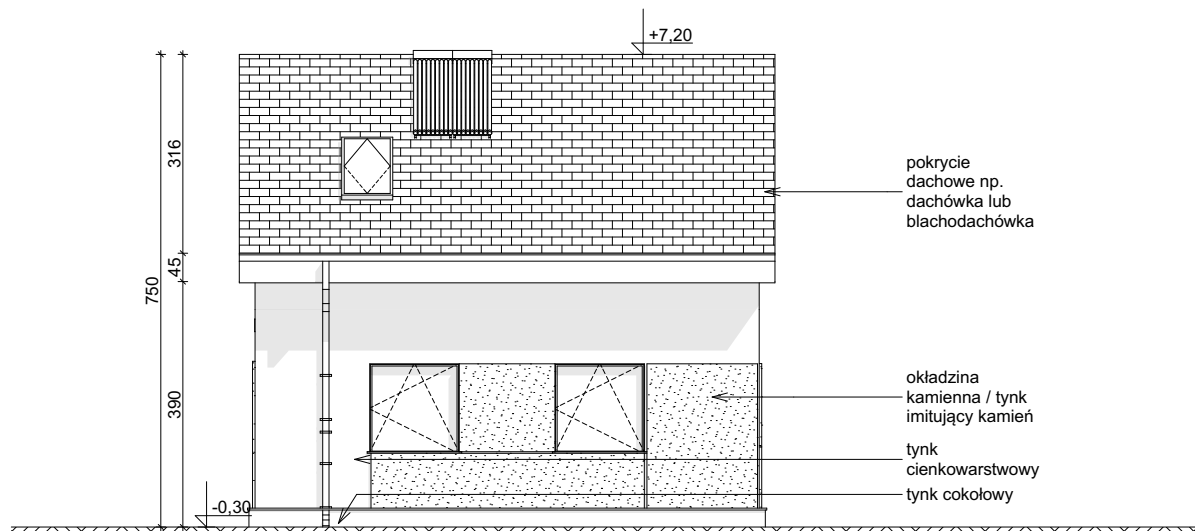
ELEWACJA OGRODOWA
