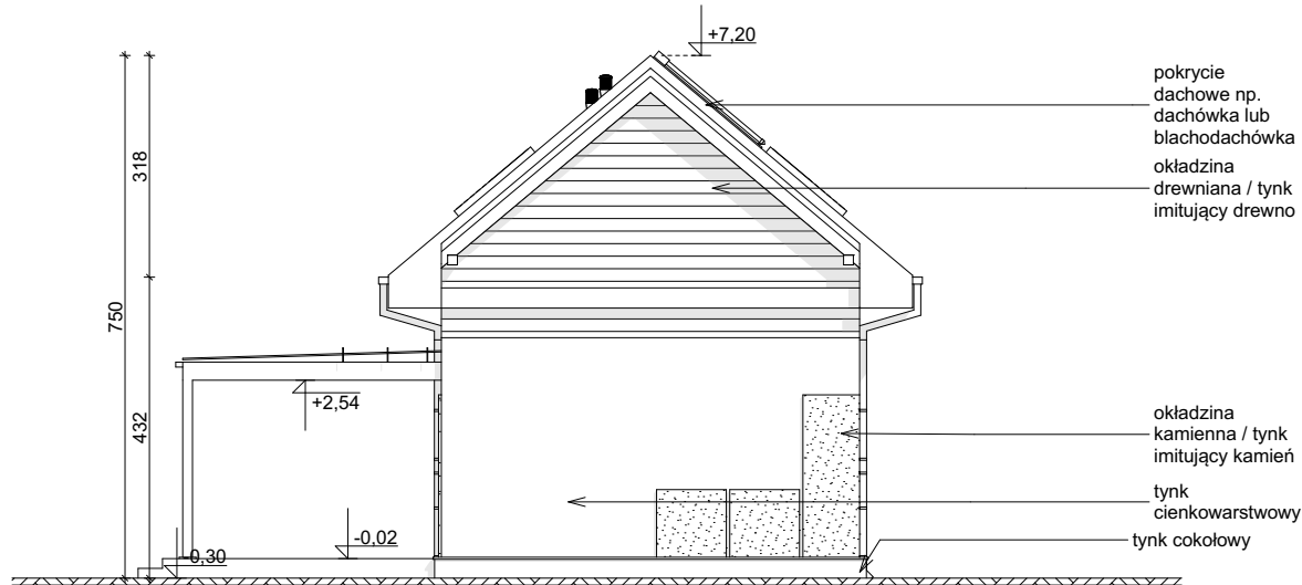
ELEWACJA BOCZNA
