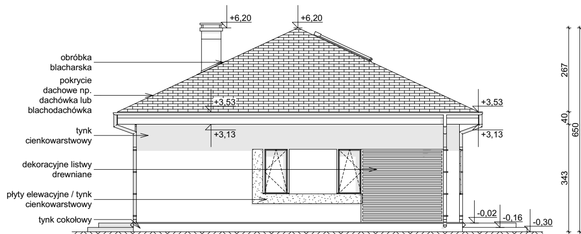
ELEWACJA BOCZNA
