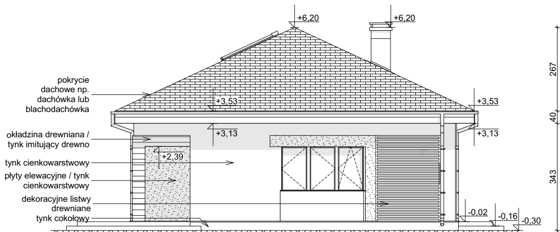
ELEWACJA BOCZNA
