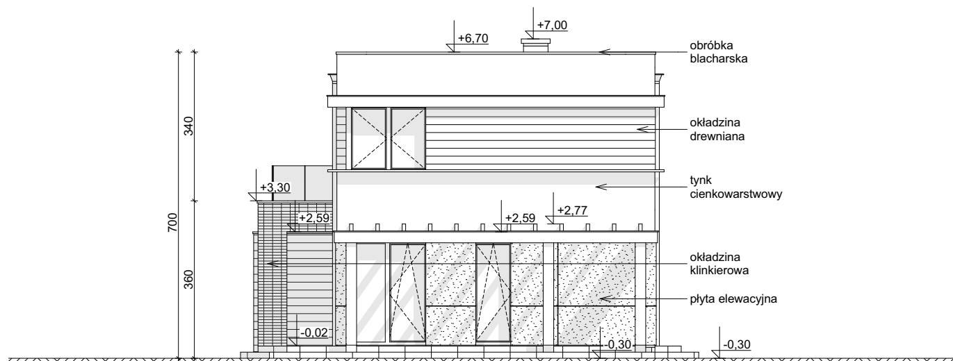
ELEWACJA BOCZNA
