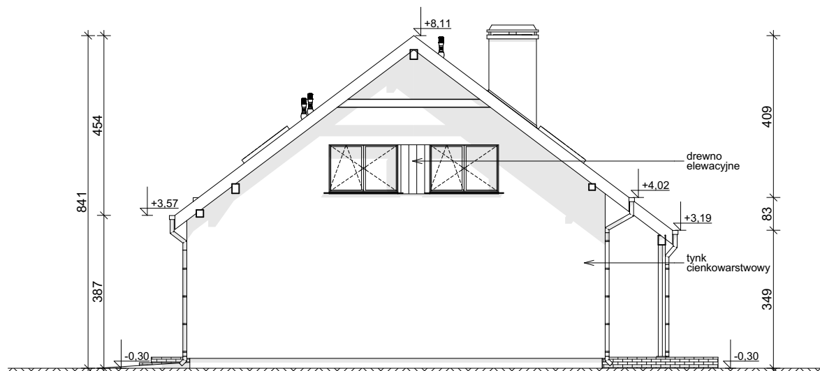
ELEWACJA BOCZNA
