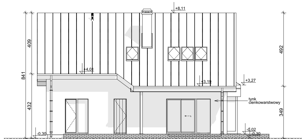
ELEWACJA OGRODOWA
