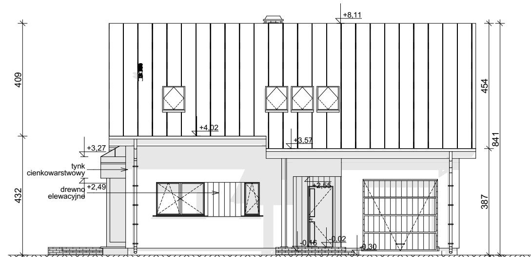
ELEWACJA FRONTOWA
