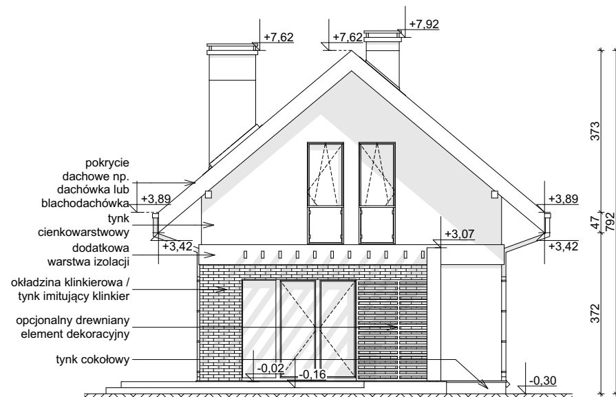
ELEWACJA OGRODOWA
