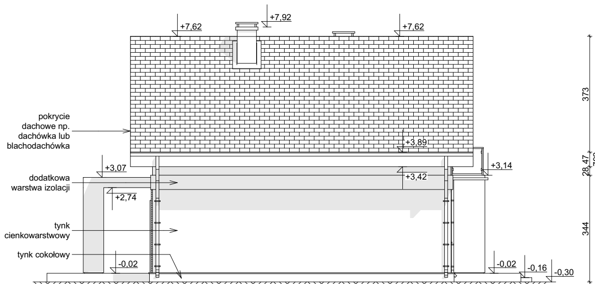
ELEWACJA BOCZNA
