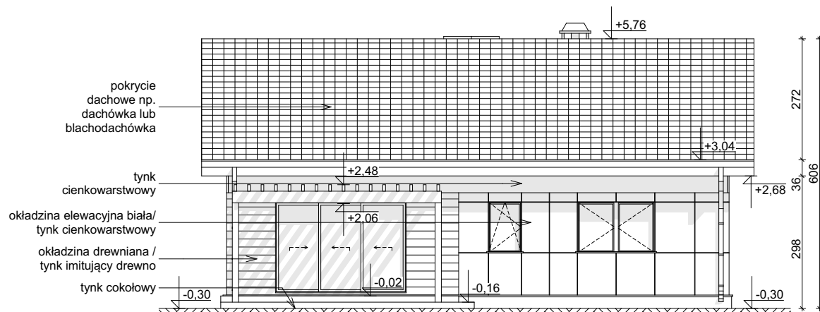
ELEWACJA OGRODOWA
