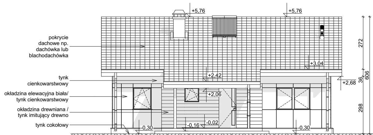
ELEWACJA FRONTOWA
