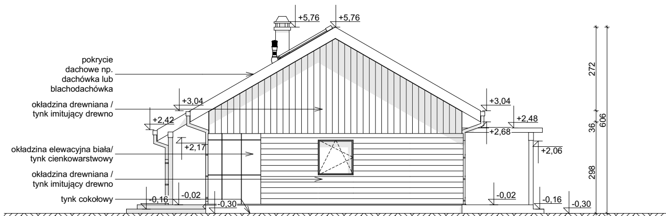
ELEWACJA BOCZNA
