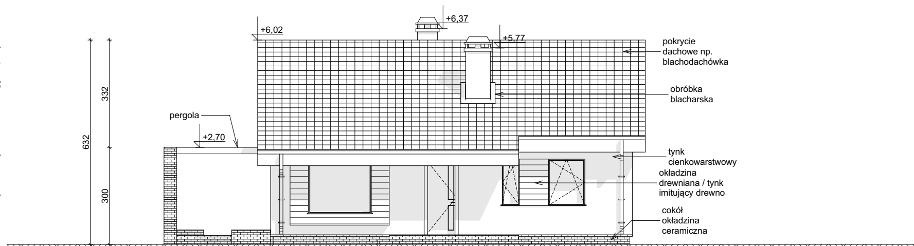
ELEWACJA FRONTOWA
