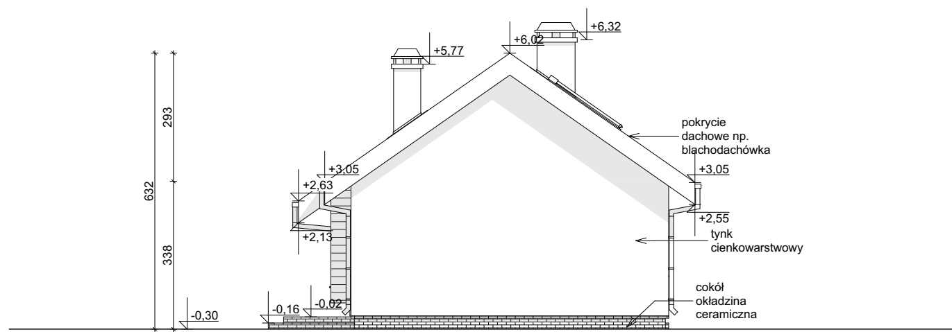
ELEWACJA BOCZNA
