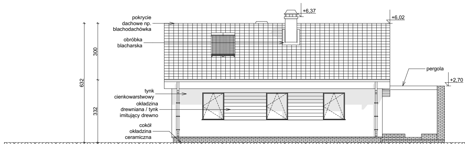
ELEWACJA OGRODOWA
