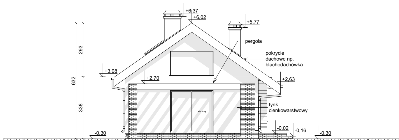
ELEWACJA BOCZNA
