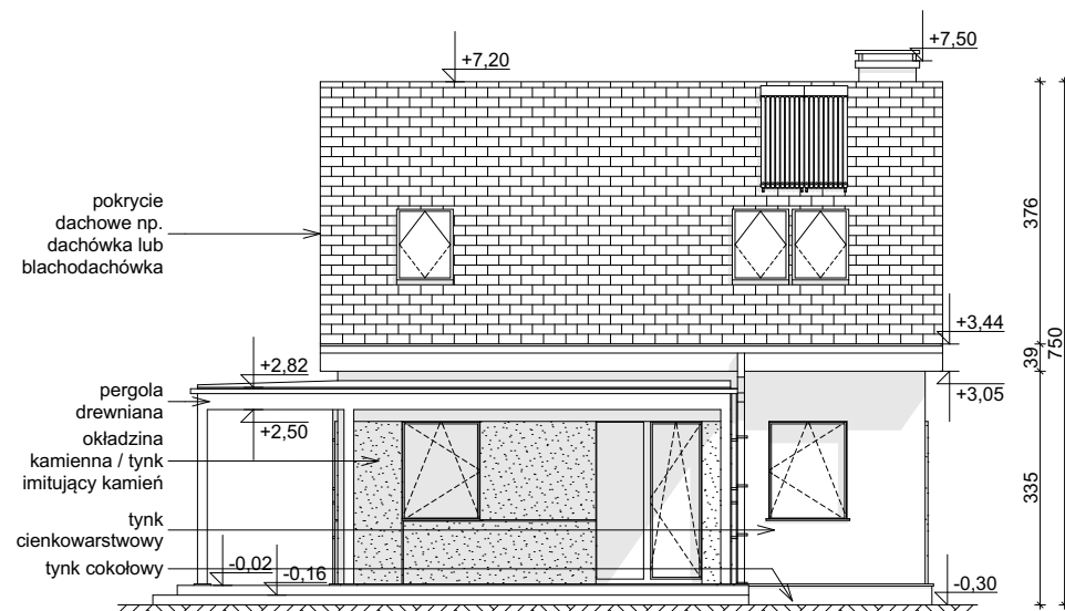
ELEWACJA OGRODOWA
