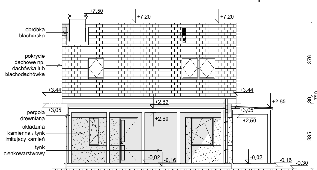
ELEWACJA FRONTOWA
