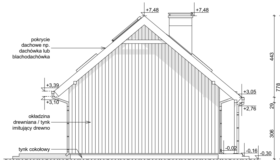
ELEWACJA BOCZNA
