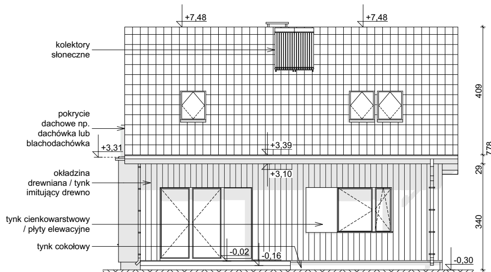
ELEWACJA OGRODOWA
