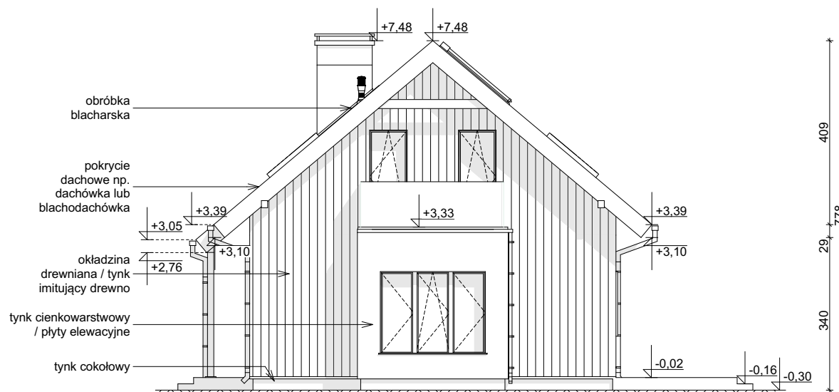
ELEWACJA BOCZNA
