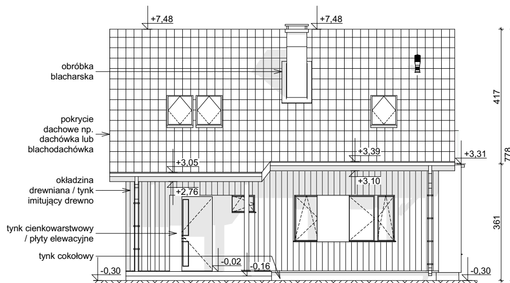
ELEWACJA FRONTOWA
