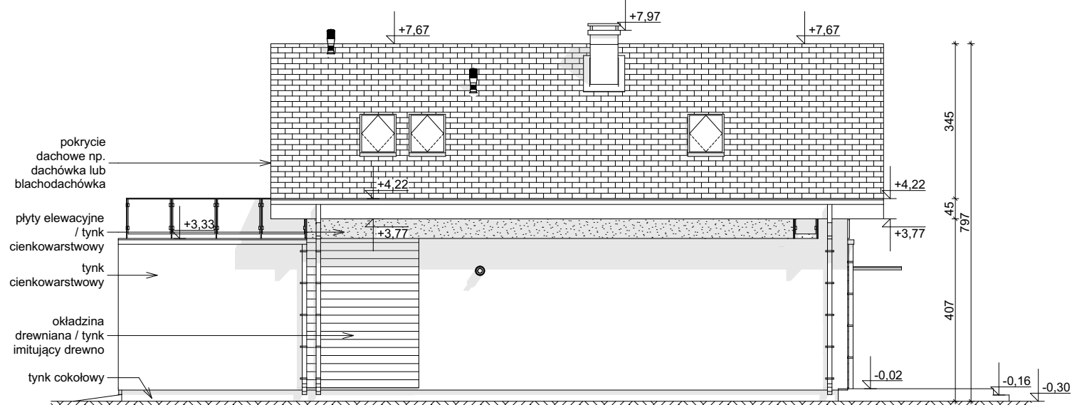
ELEWACJA BOCZNA
