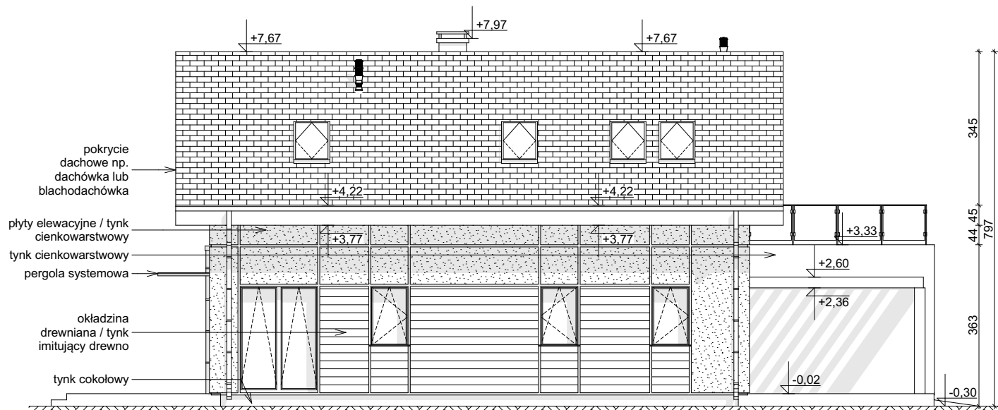
ELEWACJA BOCZNA
