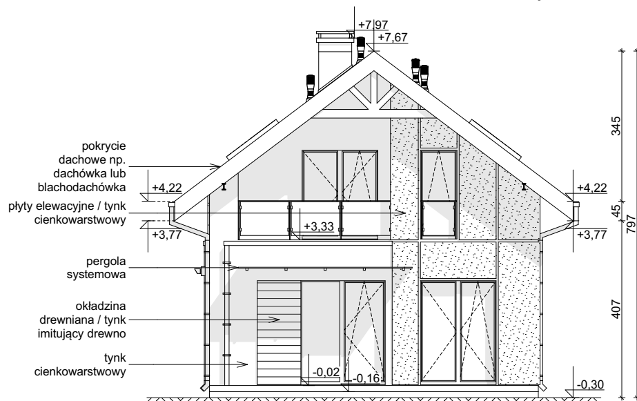
ELEWACJA OGRODOWA
