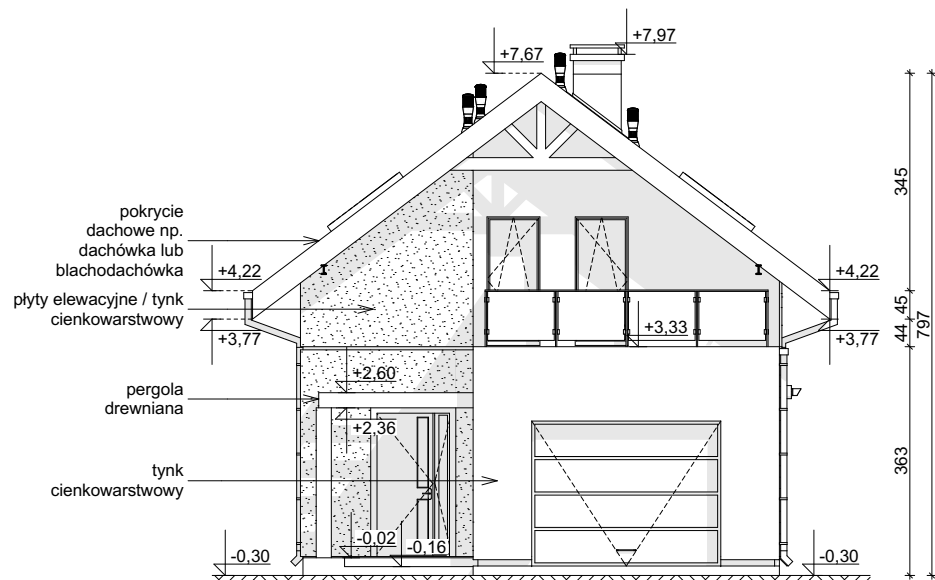
ELEWACJA FRONTOWA
