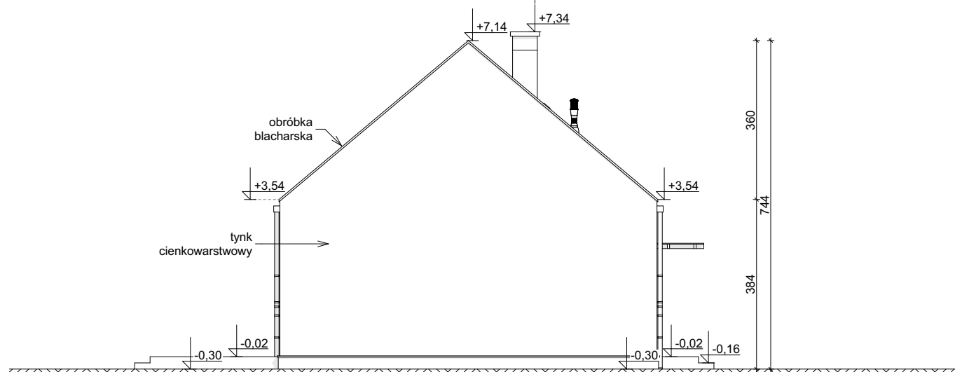
ELEWACJA BOCZNA
