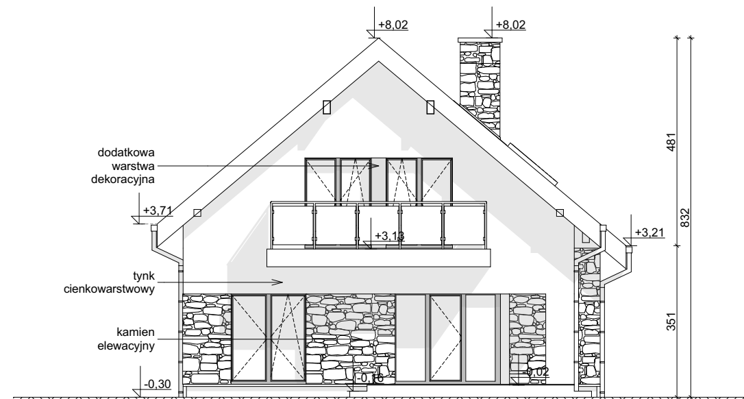
ELEWACJA OGRODOWA
