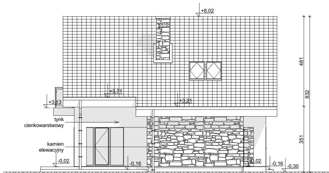
ELEWACJA BOCZNA
