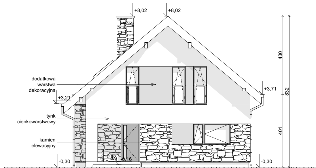
ELEWACJA FRONTOWA
