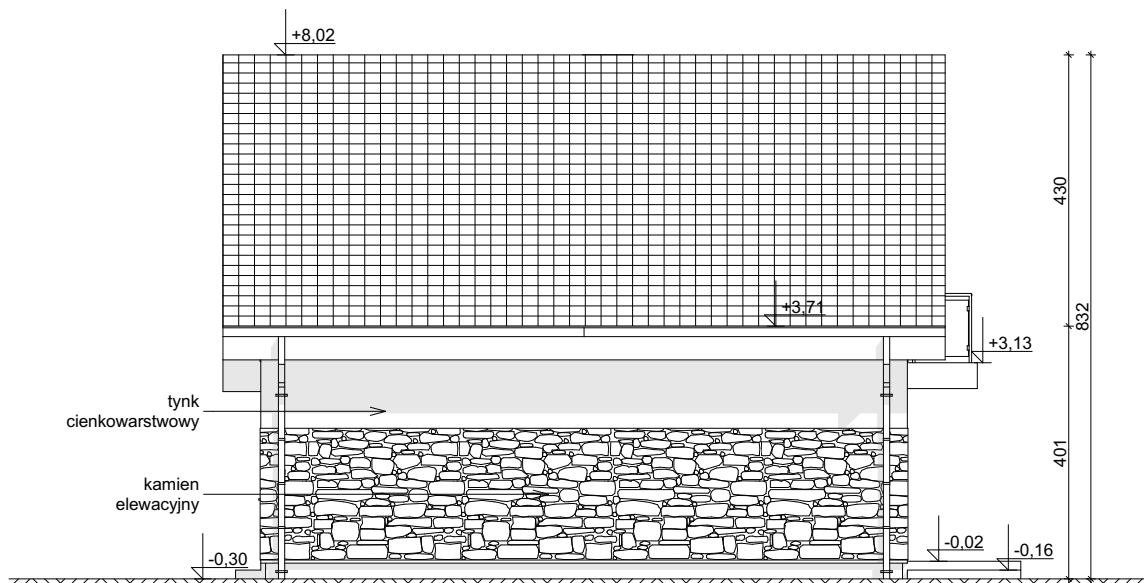
ELEWACJA BOCZNA
