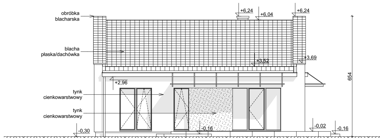
ELEWACJA OGRODOWA
