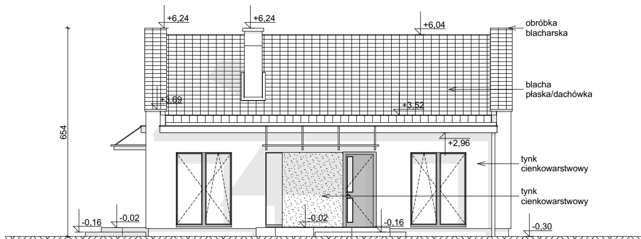
ELEWACJA FRONTOWA
