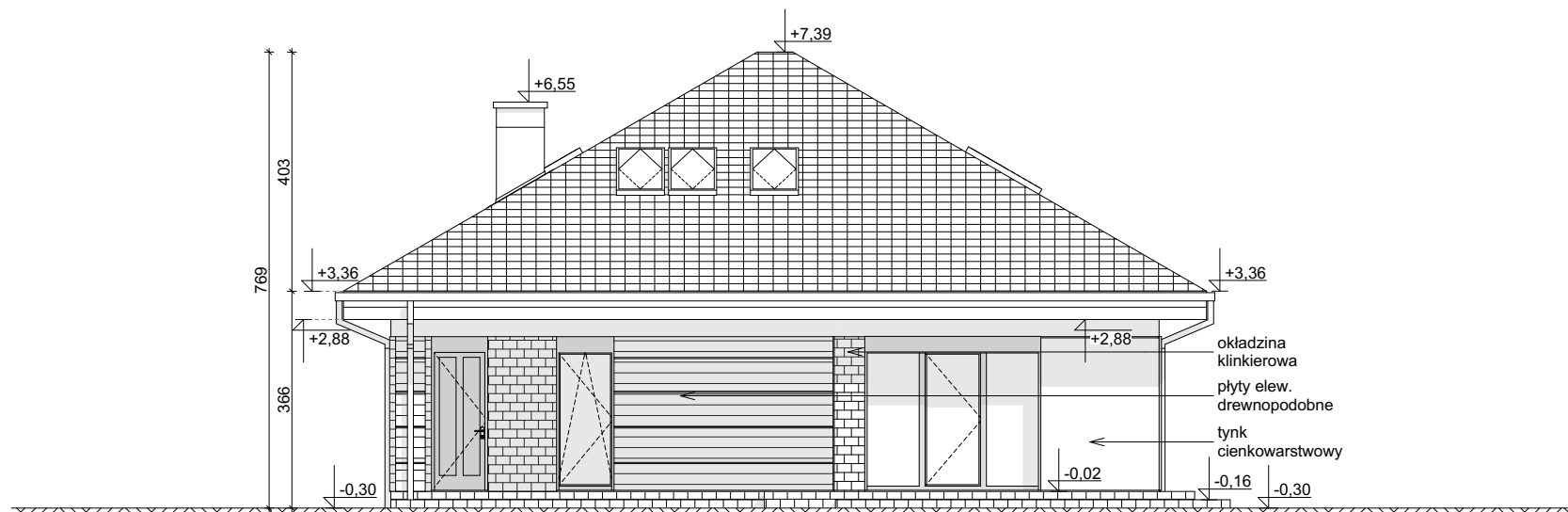
ELEWACJA OGRODOWA
