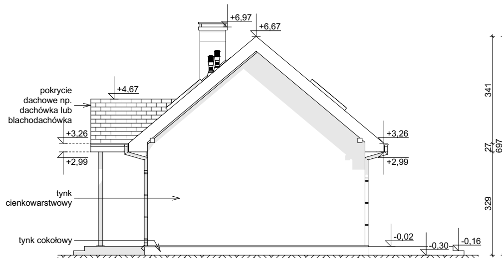
ELEWACJA BOCZNA
