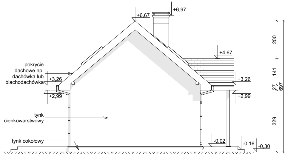
ELEWACJA BOCZNA
