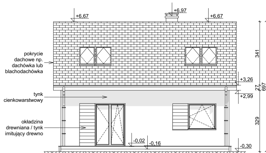
ELEWACJA OGRODOWA
