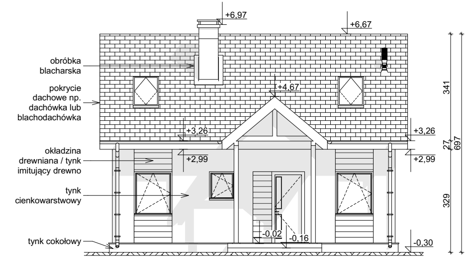
ELEWACJA FRONTOWA
