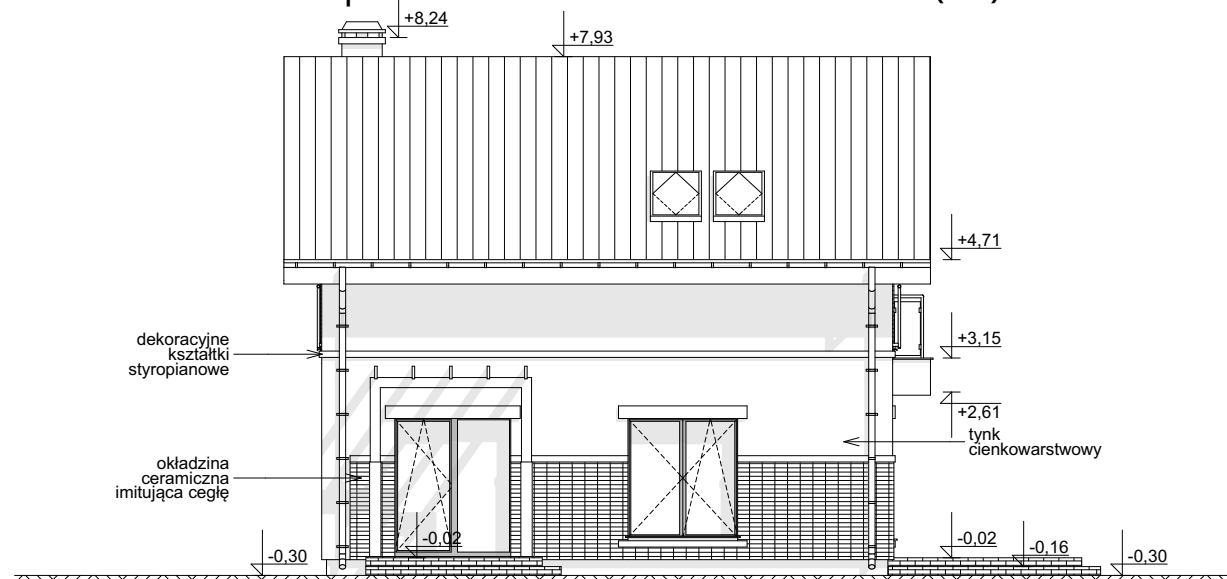
ELEWACJA OGRODOWA
