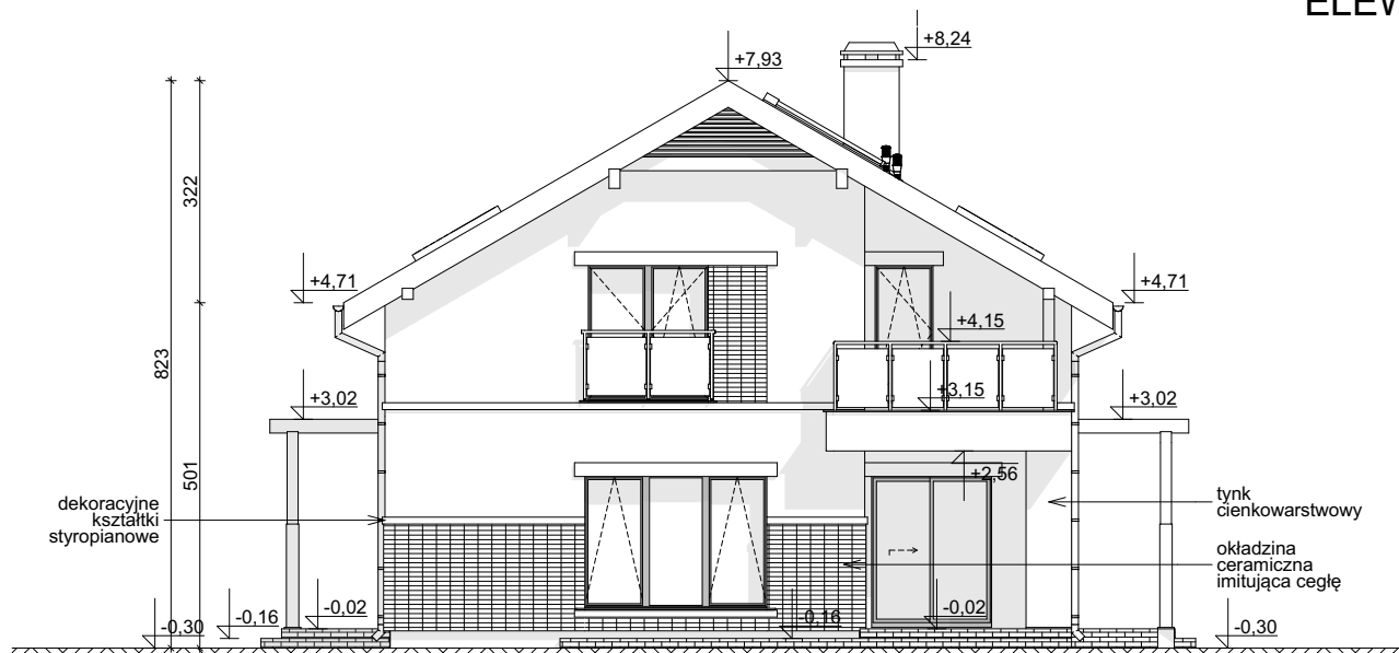
ELEWACJA BOCZNA
