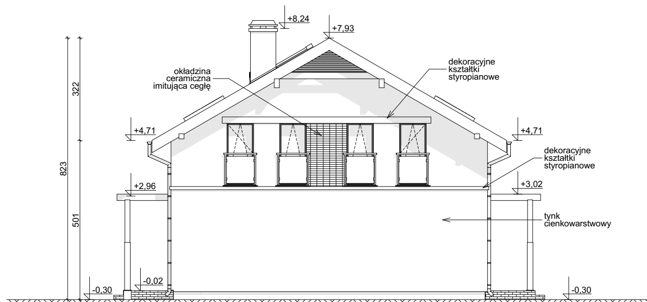
ELEWACJA BOCZNA
