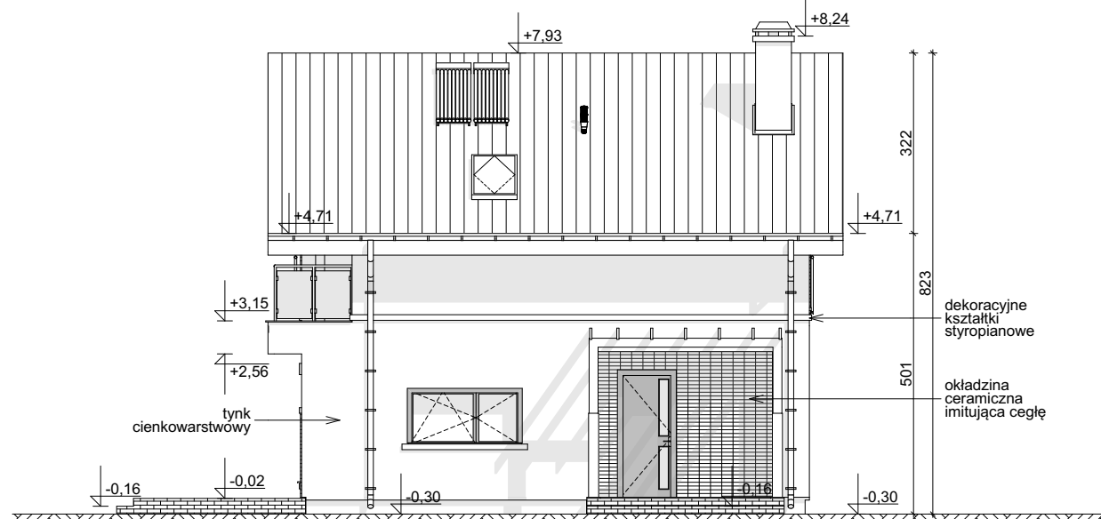
ELEWACJA FRONTOWA
