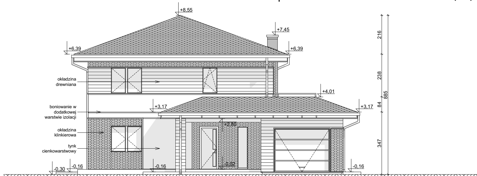
ELEWACJA FRONTOWA
