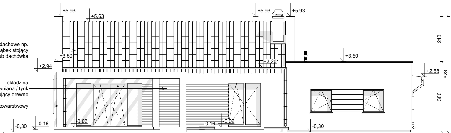
ELEWACJA OGRODOWA
