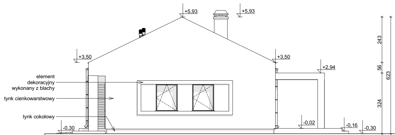
ELEWACJA BOCZNA
