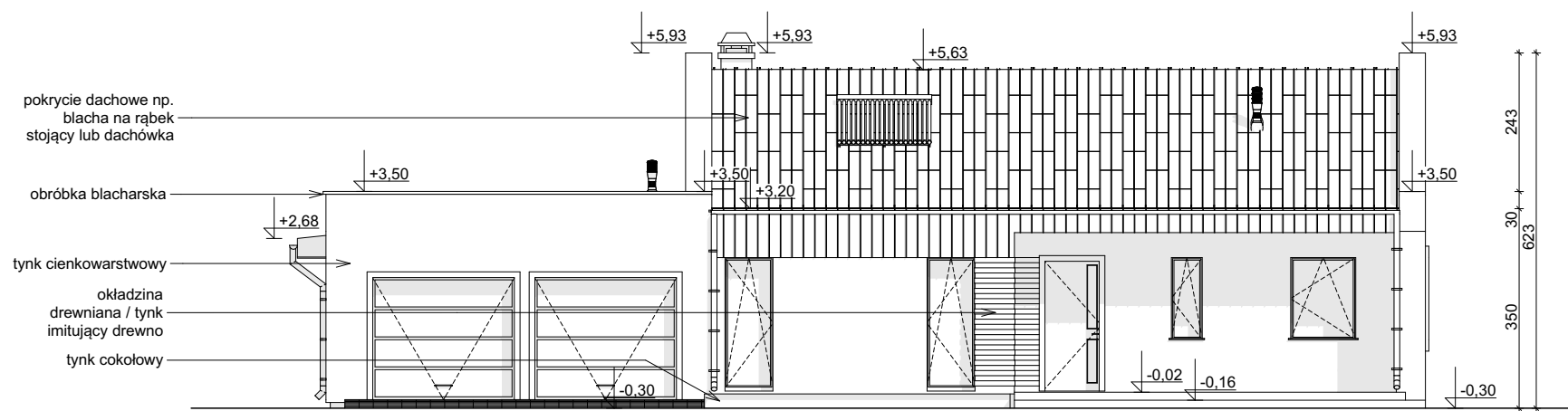
ELEWACJA FRONTOWA
