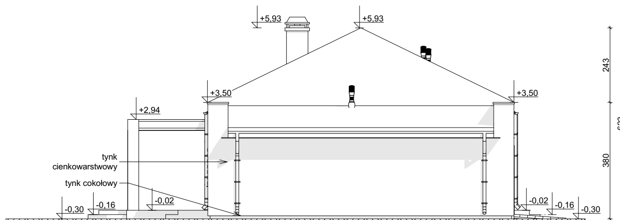
ELEWACJA BOCZNA
