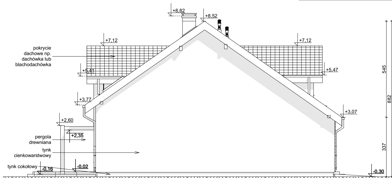
ELEWACJA BOCZNA
