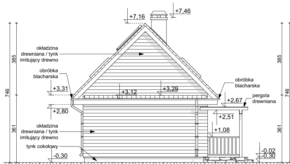
ELEWACJA BOCZNA
