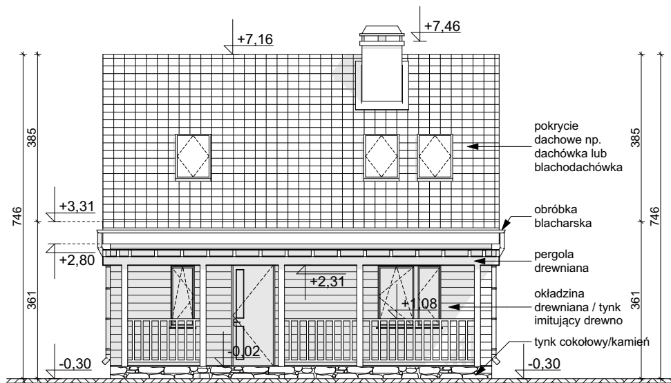
ELEWACJA FRONTOWA
