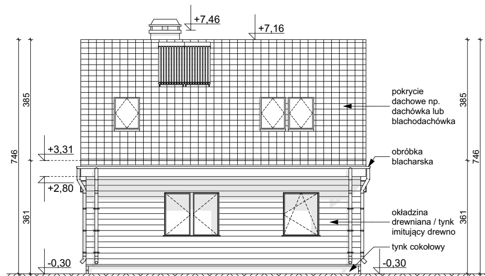
ELEWACJA OGRODOWA
