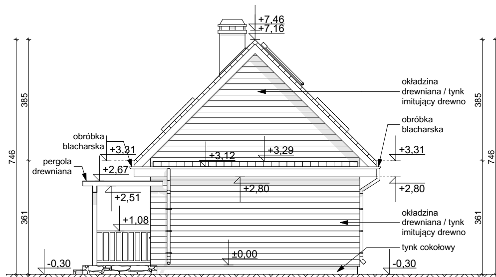
ELEWACJA BOCZNA
