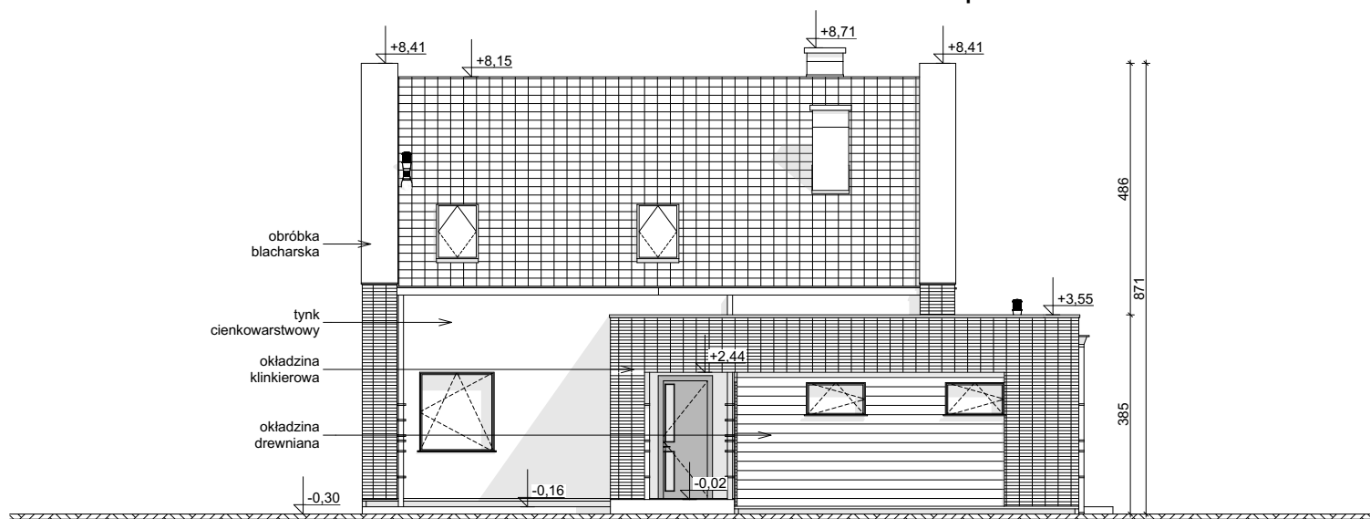
ELEWACJA FRONTOWA
