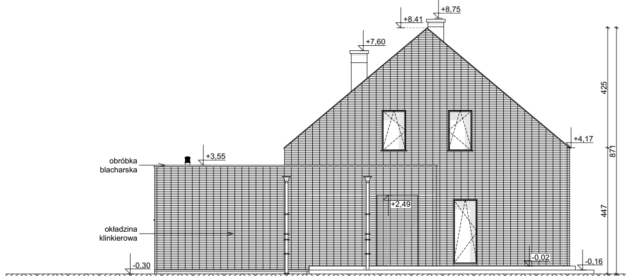
ELEWACJA BOCZNA
