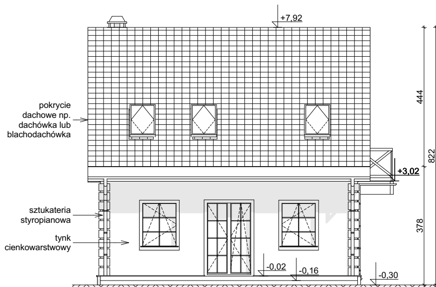
ELEWACJA OGRODOWA
