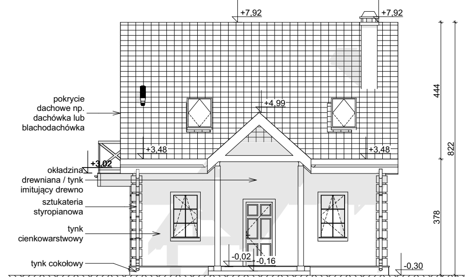
ELEWACJA FRONTOWA
