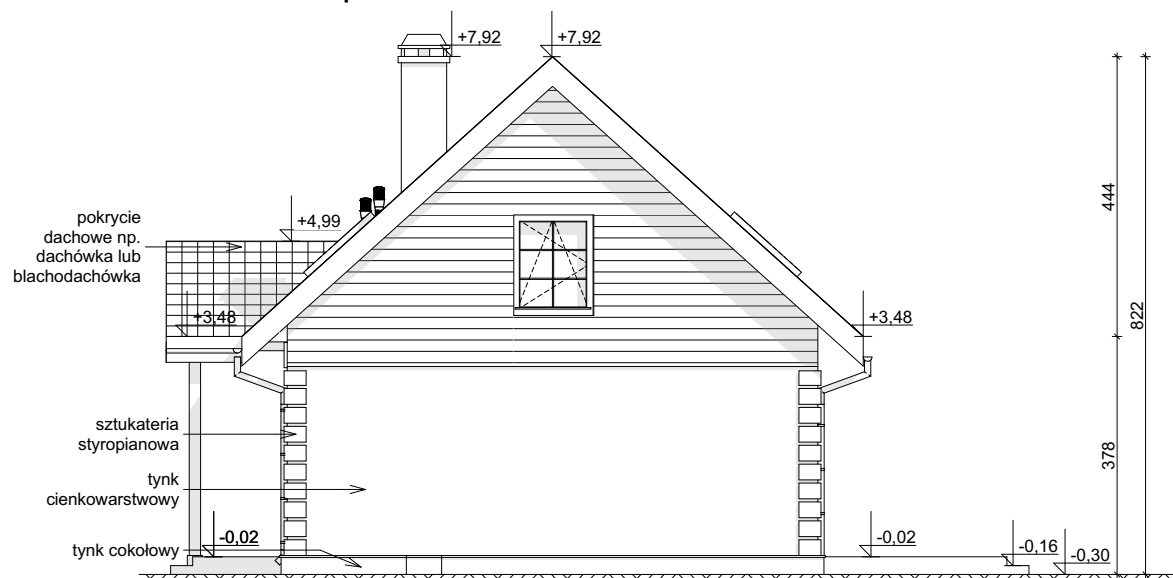
ELEWACJA BOCZNA
