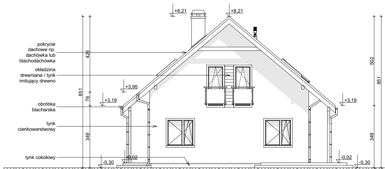
ELEWACJA BOCZNA
