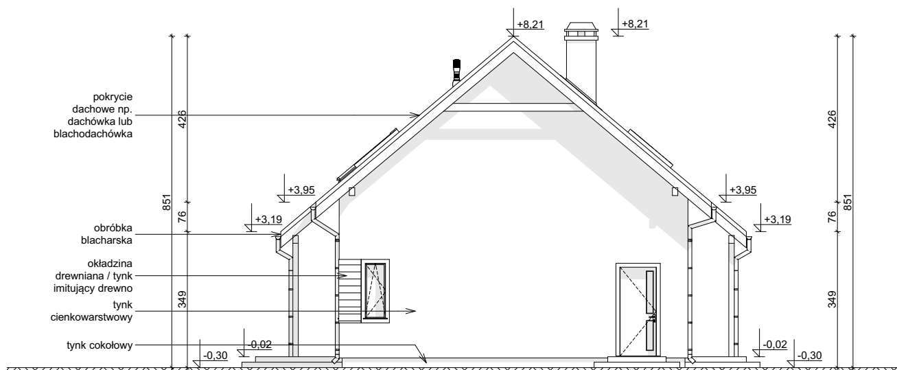
ELEWACJA BOCZNA
