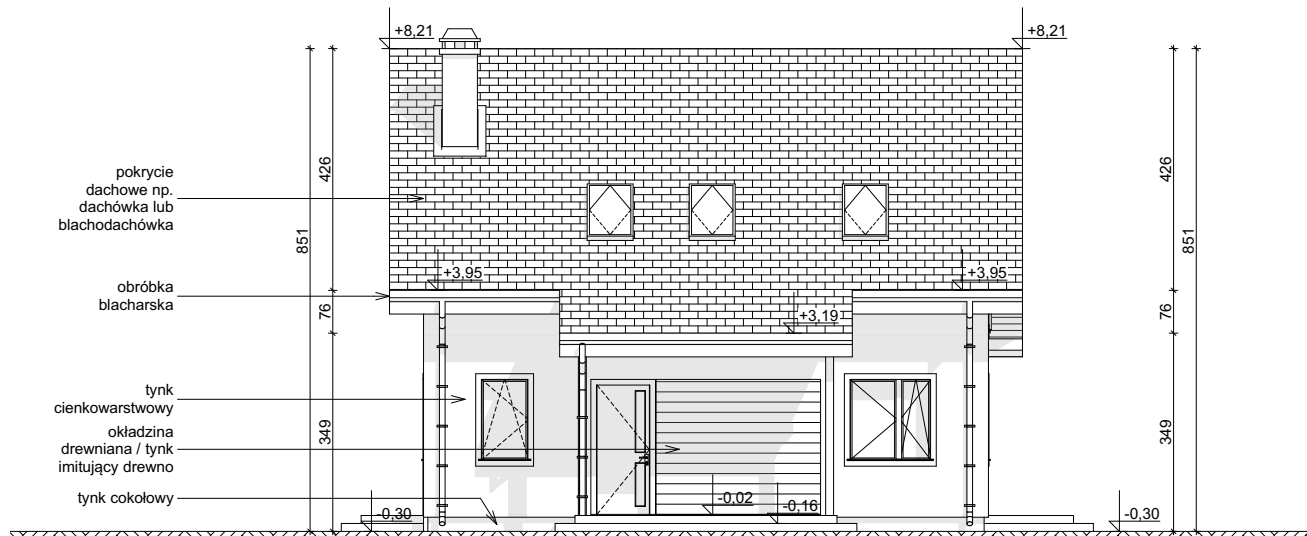
ELEWACJA FRONTOWA
