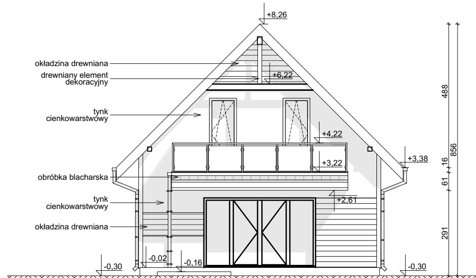
ELEWACJA OGRODOWA
