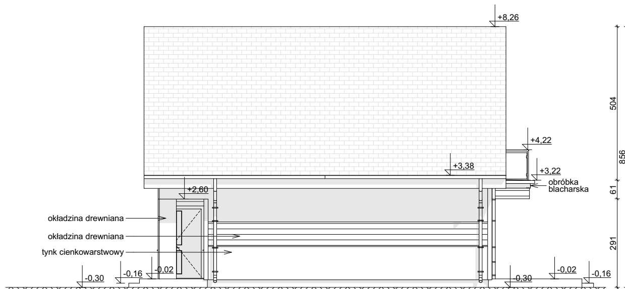
ELEWACJA BOCZNA
