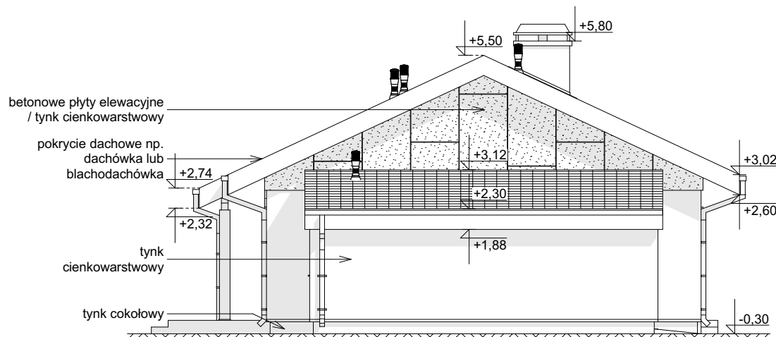
ELEWACJA BOCZNA
