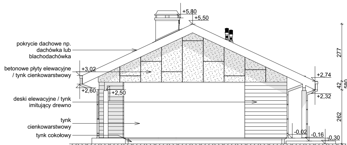
ELEWACJA BOCZNA
