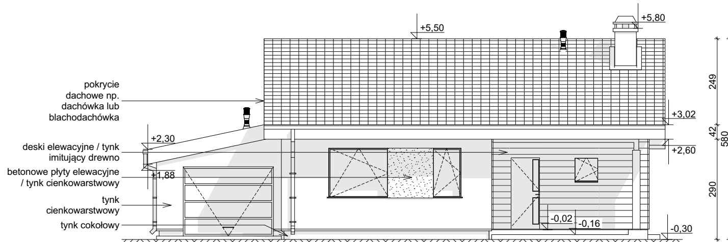
ELEWACJA FRONTOWA
