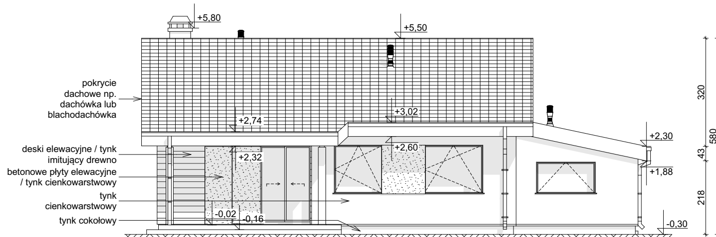
ELEWACJA OGRODOWA
