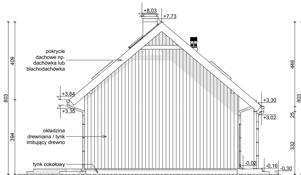
ELEWACJA BOCZNA
