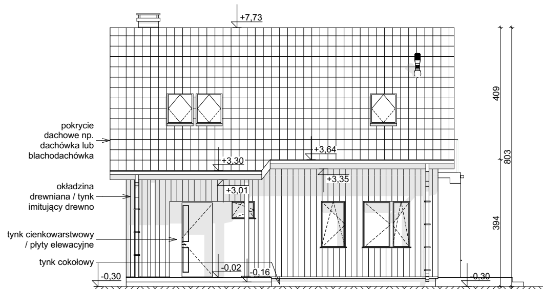
ELEWACJA FRONTOWA
